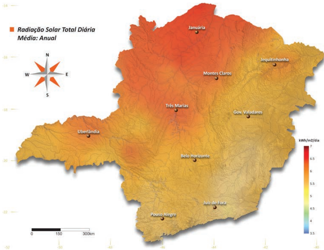
Figura 56A . Irradiação solar diária, média anual: período 2008-2010
