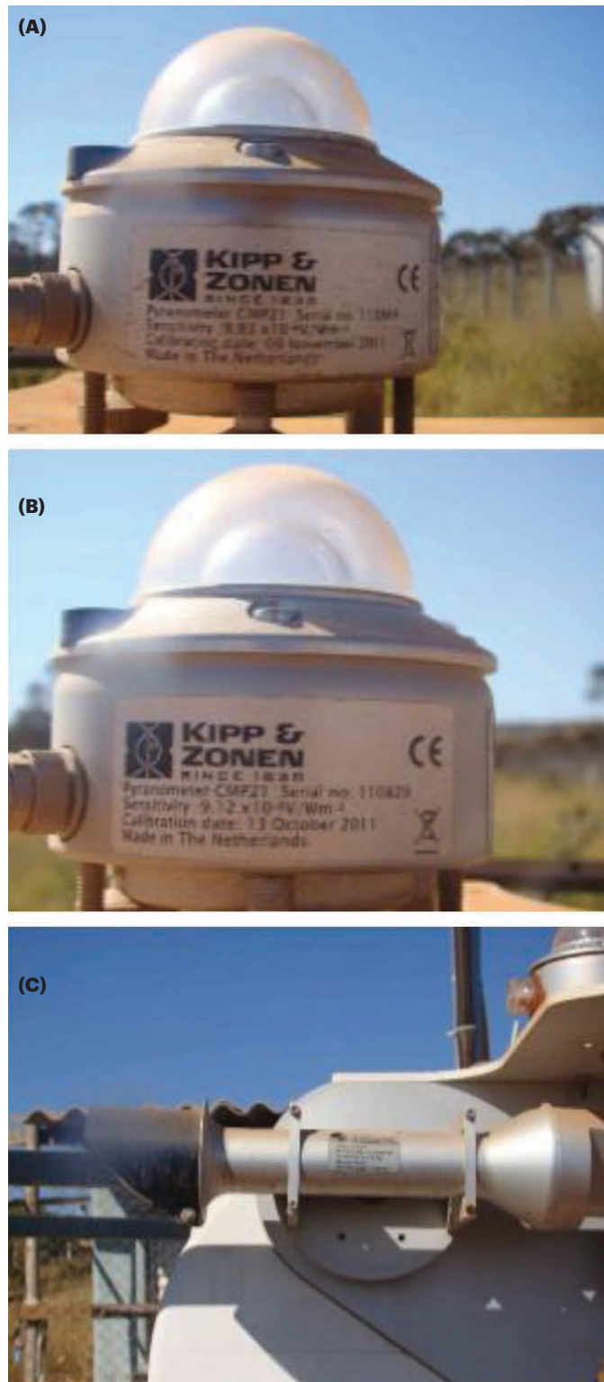
Figura 24 . (A) detalhe piranômetro CMP 21, radiação global; (B) detalhe piranômetro CMP 21, radiação difusa; (C) detalhe piroheliômetro CHP1, radiação direta. Todos instalados a 1,70 metros em relação ao solo.
