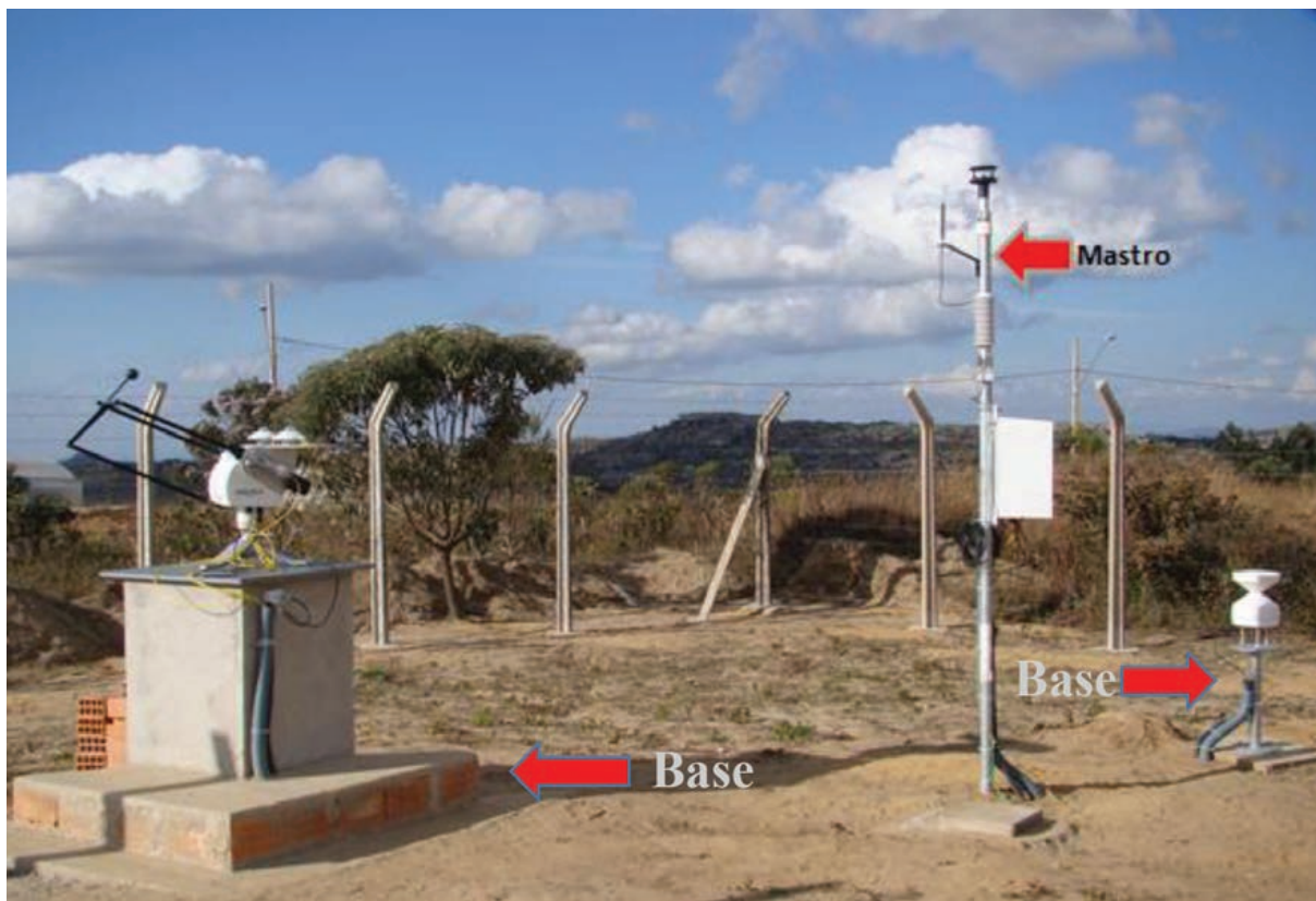
Figura 30 . Estação Solarimétrica de Diamantina.
