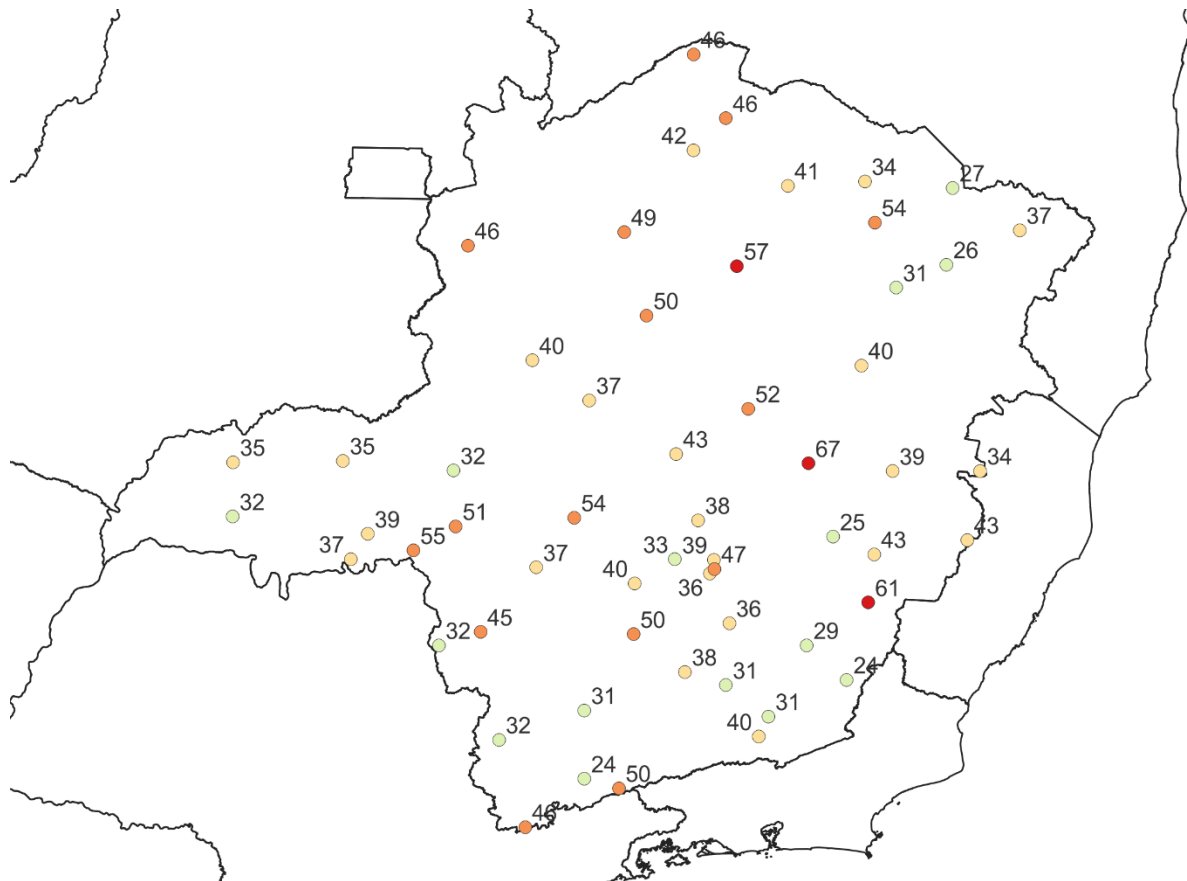
Figura 4 – Rajadas de vento máximas registradas entre os dias 08 e 12 de fevereiro de 2022. Fonte: INMET
