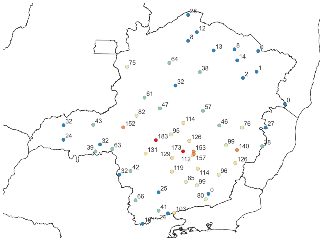
Figura 5b - Pluviometria acumulada entre os dias 08 e 12 de fevereiro de 2022. Fonte dos dados: INMET.
