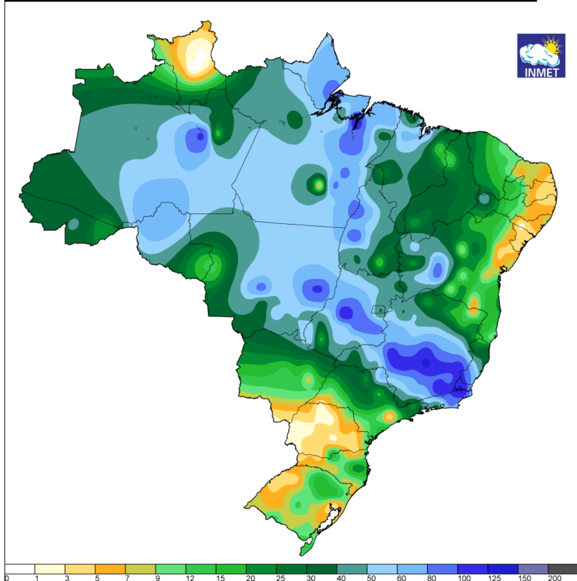
Figura 5a - Pluviometria acumulada entre os dias 08 e 12 de fevereiro de 2022. Fonte: INMET.
