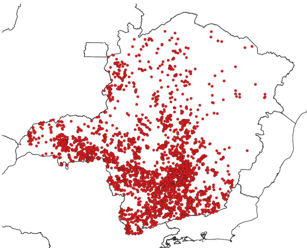
Figura 3 - Localização dos raios registrados entre os dias 08 e 12 de fevereiro de 2022. Fonte: RINDAT
