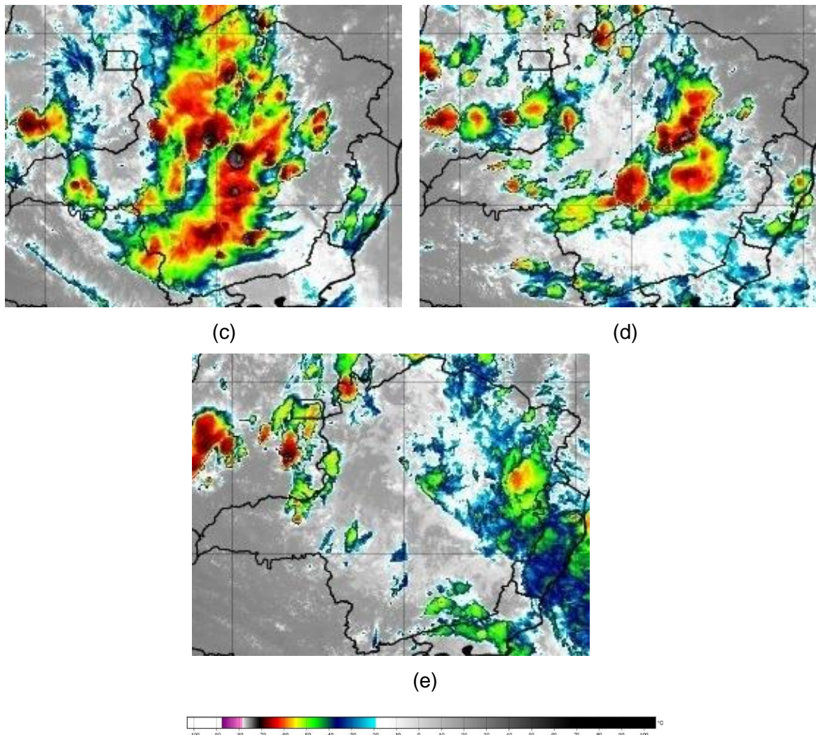
Figura 2 – Seleção de Imagem de Satélite dos dias 08 as 18:00 (a), 09 as 19:00 (b), 10 as 17:00 (c), 11 as 17:00 e 12 as 19:00 de fevereiro de 2022 (Horário Local). Fonte: INPE.
