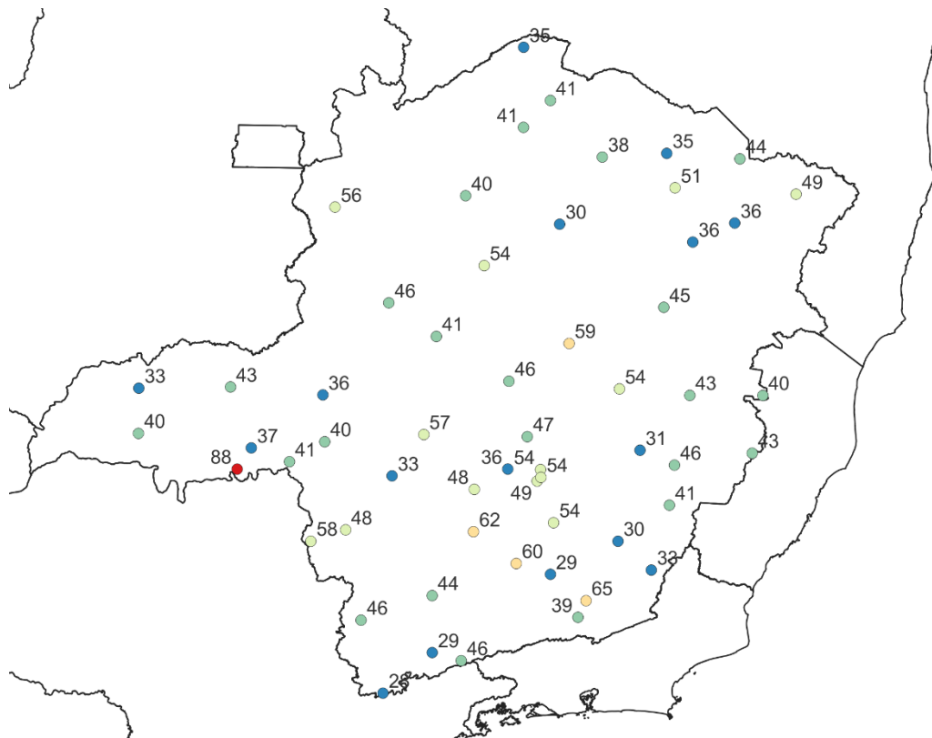
Figura 4 – Rajadas de vento máximas registradas entre os dias 16 e 20 de fevereiro de 2022. Fonte: INMET
