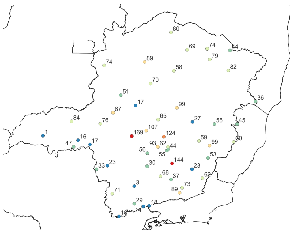
Figura 5b - Pluviometria acumulada entre os dias 16 e 20 de fevereiro de 2022. Fonte dos dados: INMET.
