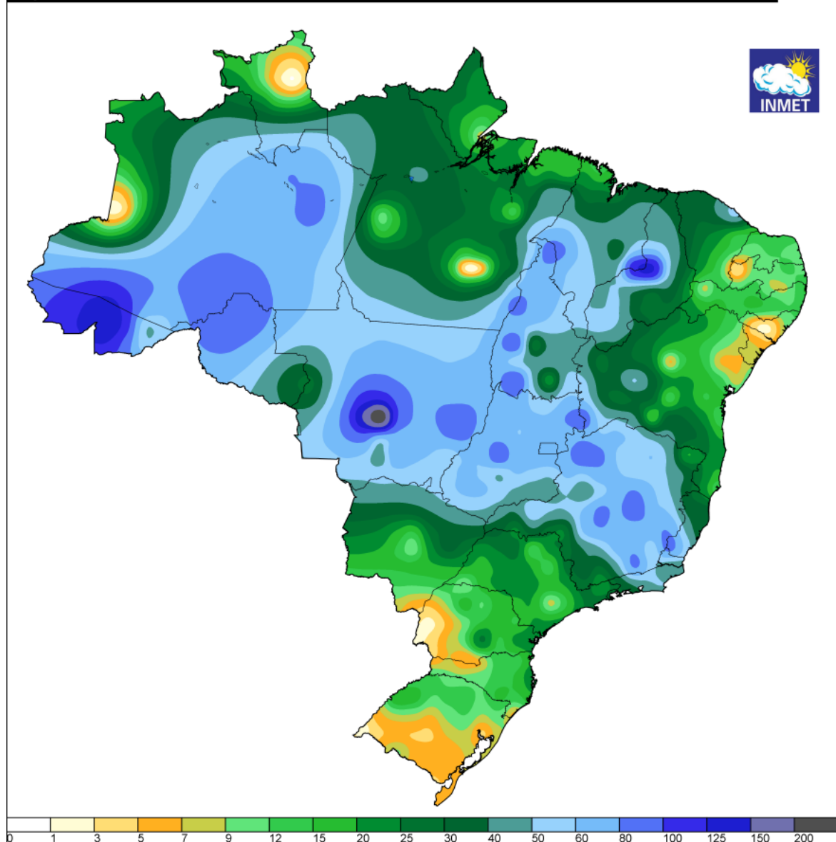
Figura 5a - Pluviometria acumulada entre os dias 16 e 20 de fevereiro de 2022. Fonte: INMET.
