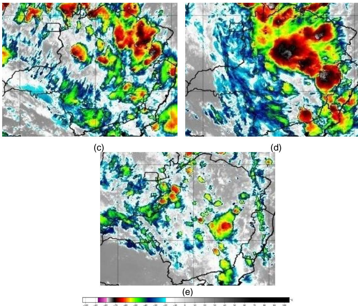
Figura 2 – Seleção de Imagem de Satélite dos dias 16 as 19:00 (c), 17 as 17:00, 18 as 17:00, 19 às 18:00 e 20 de fevereiro de 2022. Fonte: INPE.
