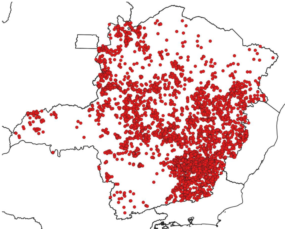
Figura 3 - Localização dos raios registrados entre os dias 16 e 20 de fevereiro de 2022. Fonte: RINDAT
