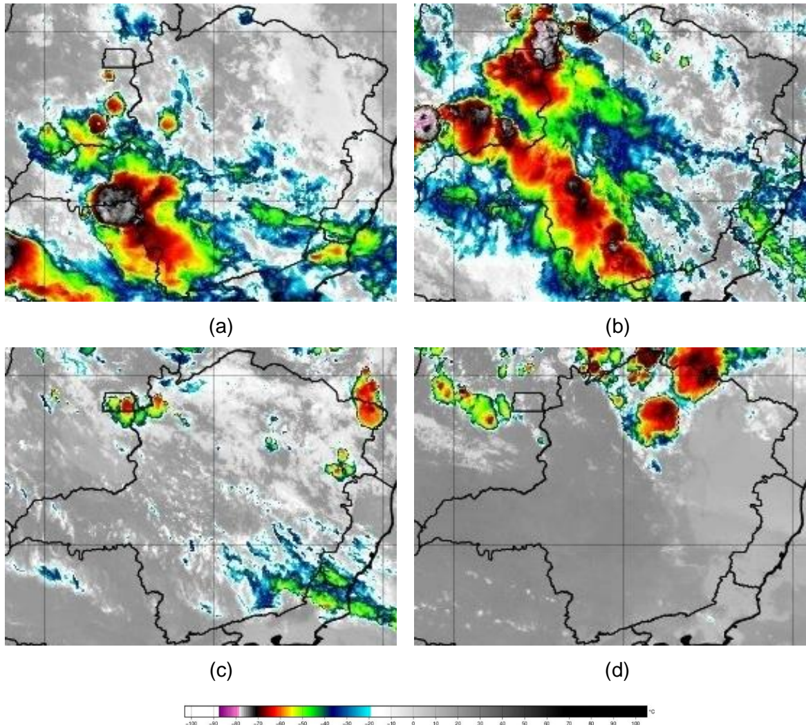
Figura 2 – Seleção de Imagem de Satélite dos dias 21 (a), 22 (b), 23 (c) e 24 (d) de setembro de 2022. Fonte: INPE.
