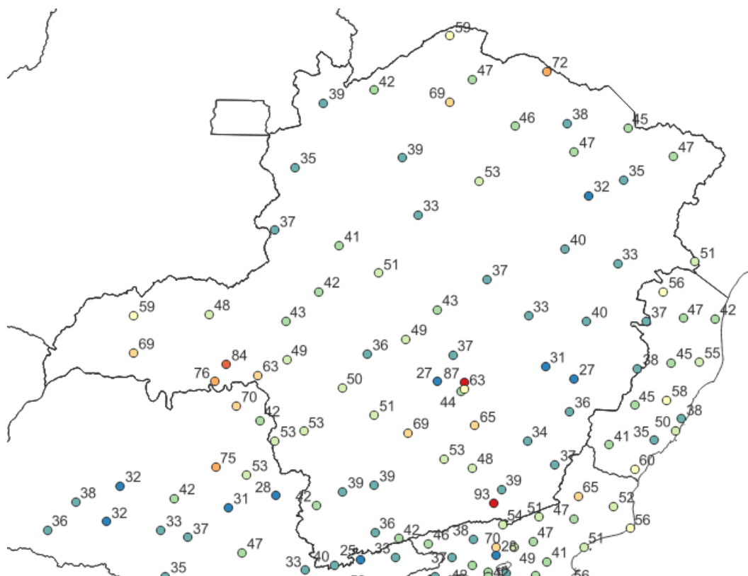
Figura 4 – Rajadas de vento máximas registradas entre os dias 21 e 24 de setembro de 2022. Fonte: INMET
