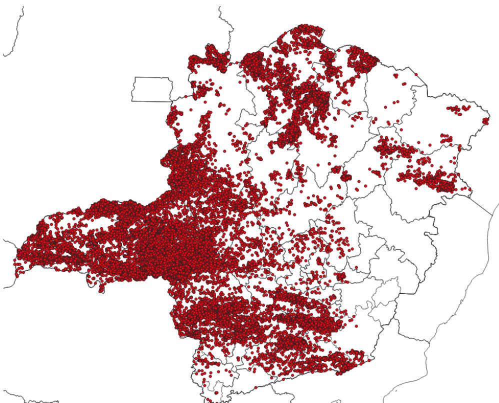
Figura 3 - Localização dos raios registrados entre os dias 21 e 24 de setembro de 2022. Fonte: RINDAT
