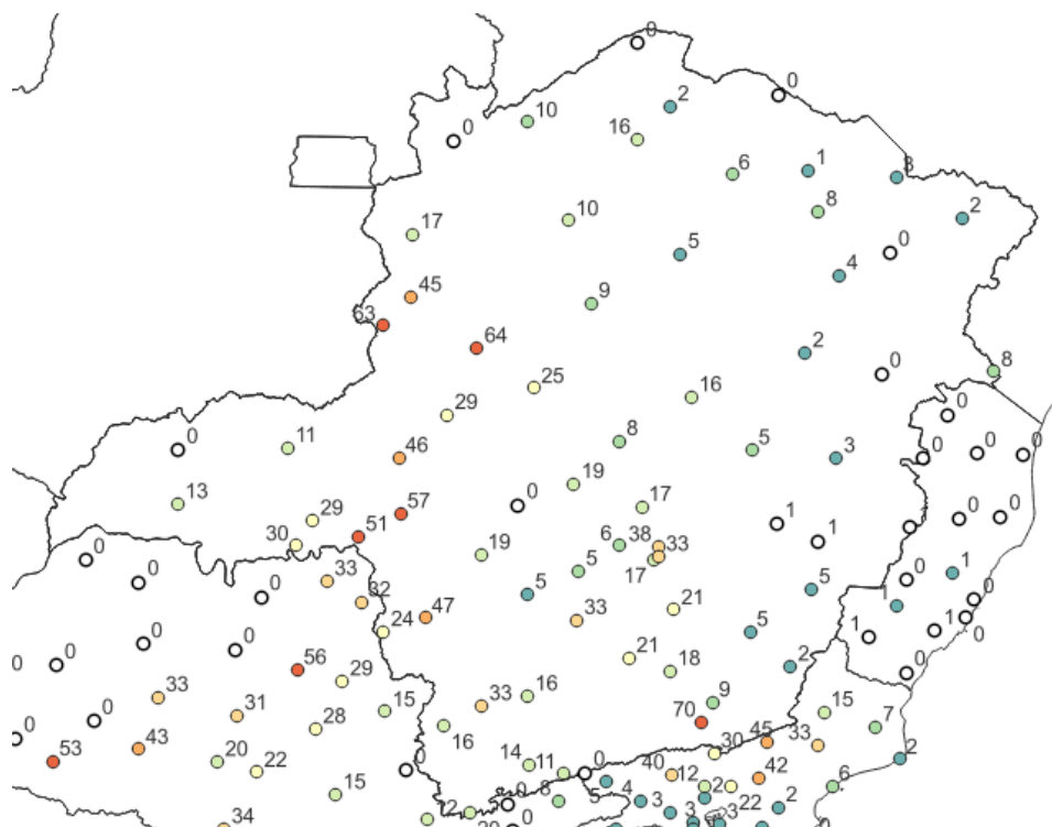
Figura 5b - Pluviometria acumulada entre os dias 21 e 24 de setembro de 2022. Fonte dos dados: INMET.
