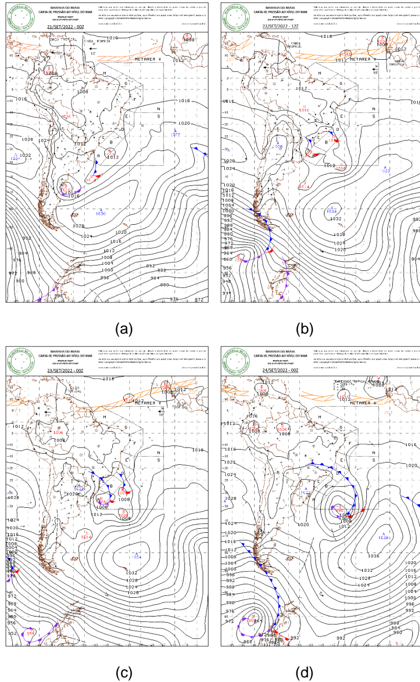
Figura 1 - Carta Sinótica em superfície dos dias 21 (a), 22 (b), 23 (c) e 24 de setembro de 2022. Fonte: Marinha do Brasil.
