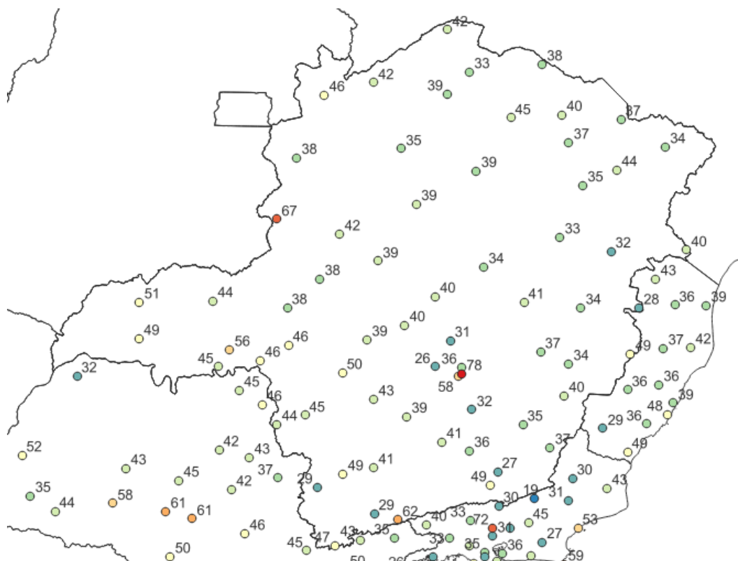
Figura 4 – Rajadas de vento máximas registradas entre os dias 26 e 30 de setembro de 2022. Fonte: INMET
