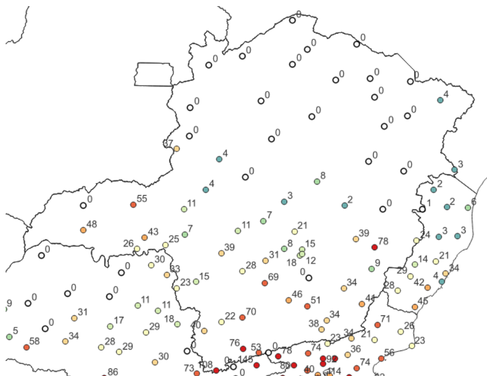
Figura 5b - Pluviometria acumulada entre os dias 26 e 30 de setembro de 2022. Fonte dos dados: INMET.
