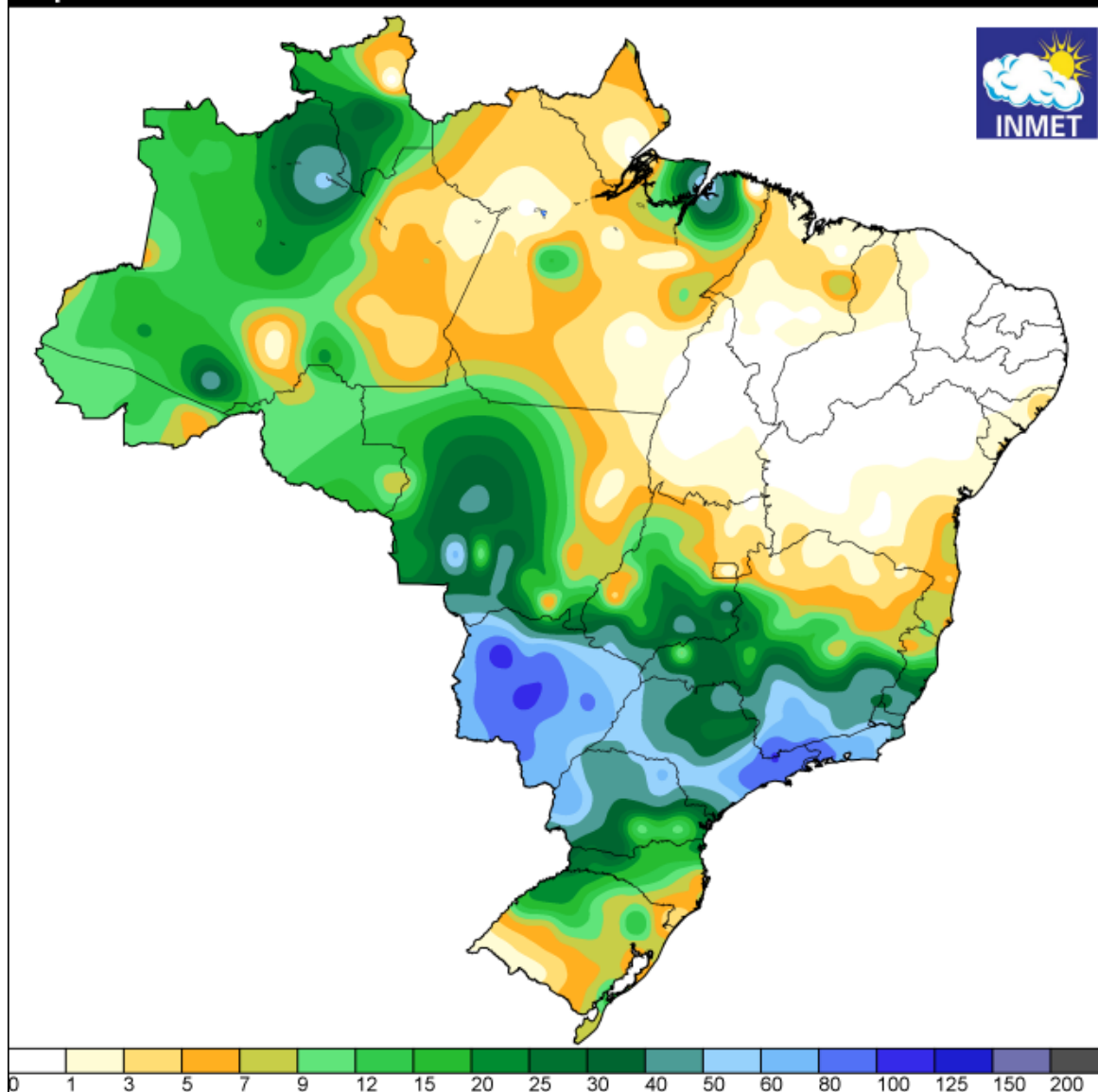
Figura 5a - Pluviometria acumulada entre os dias 20 e 24 de setembro de 2022. Fonte: INMET.
