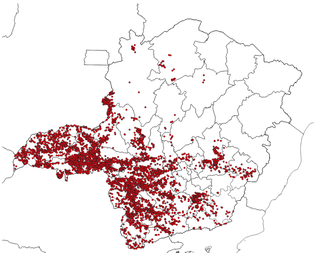
Figura 3 - Localização dos raios registrados entre os dias 26 e 30 de setembro de 2022. Fonte: RINDAT
