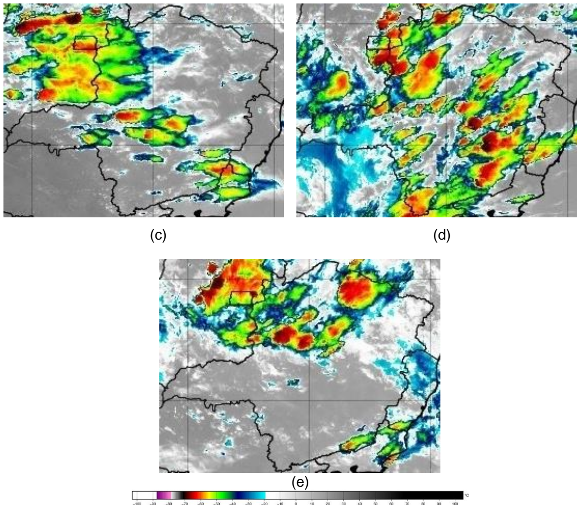
Figura 2 – Seleção de Imagem de Satélite dos dias 08 (a), 09 (b), 10 (c), 11 (d) e 12 (e) de novembro de 2022. Fonte: INPE.
