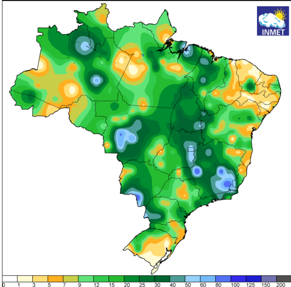
Figura 5a - Pluviometria acumulada (mm) entre os dias 08 e 12 de novembro de 2022. Fonte: INMET.
