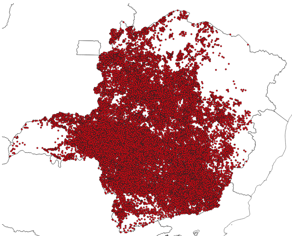
Figura 3 - Localização dos raios registrados entre os dias 08 e 12 de novembro de 2022. Fonte: RINDAT
