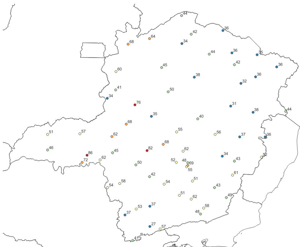
Figura 4 – Rajadas de vento máximas (Km/h) registradas entre os dias 08 e 12 de novembro de 2022. Fonte: INMET
