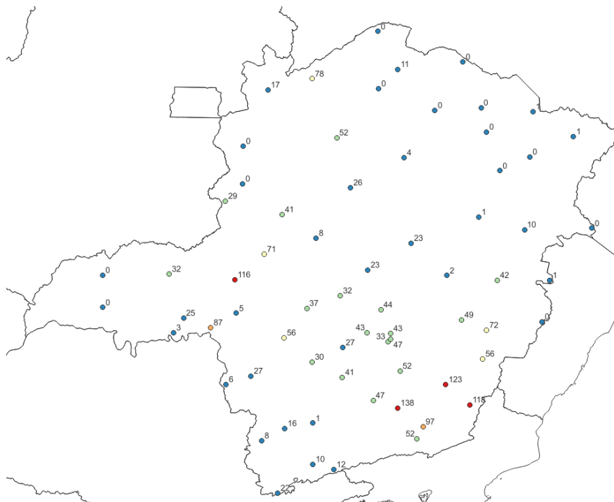
Figura 5b - Pluviometria acumulada (mm) entre os dias 08 e 12 de novembro de 2022. Fonte dos dados: INMET.
