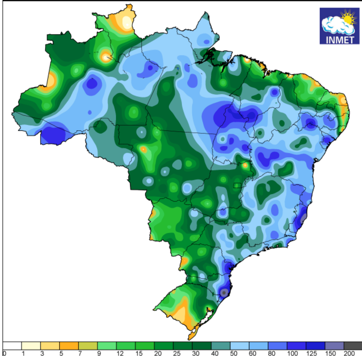
Figura 5a - Pluviometria acumulada (mm) entre os dias 28/11 e 02/12 de 2022. Fonte: INMET.
