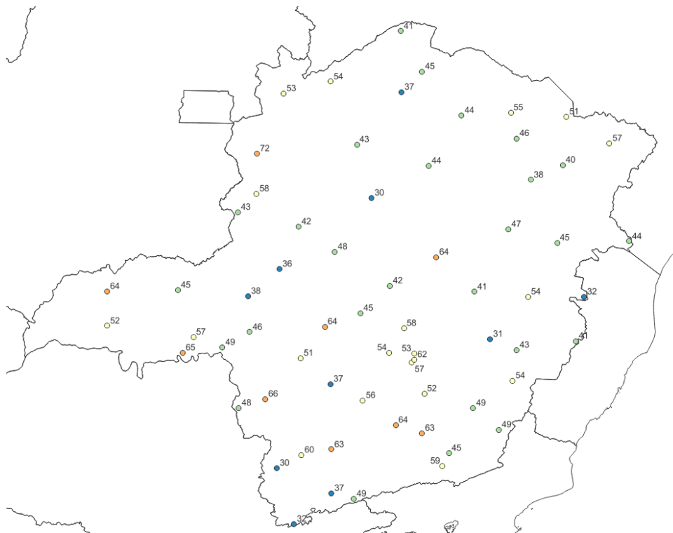
Figura 4 – Rajadas de vento (Km/h) máximas registradas entre os dias 28/11 e 02/12 de novembro de 2022. Fonte: INMET
