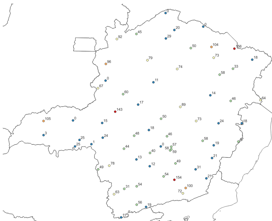
Figura 5b - Pluviometria acumulada entre os dias 28/11 e 02/12 de 2022. Fonte dos dados: INMET.
