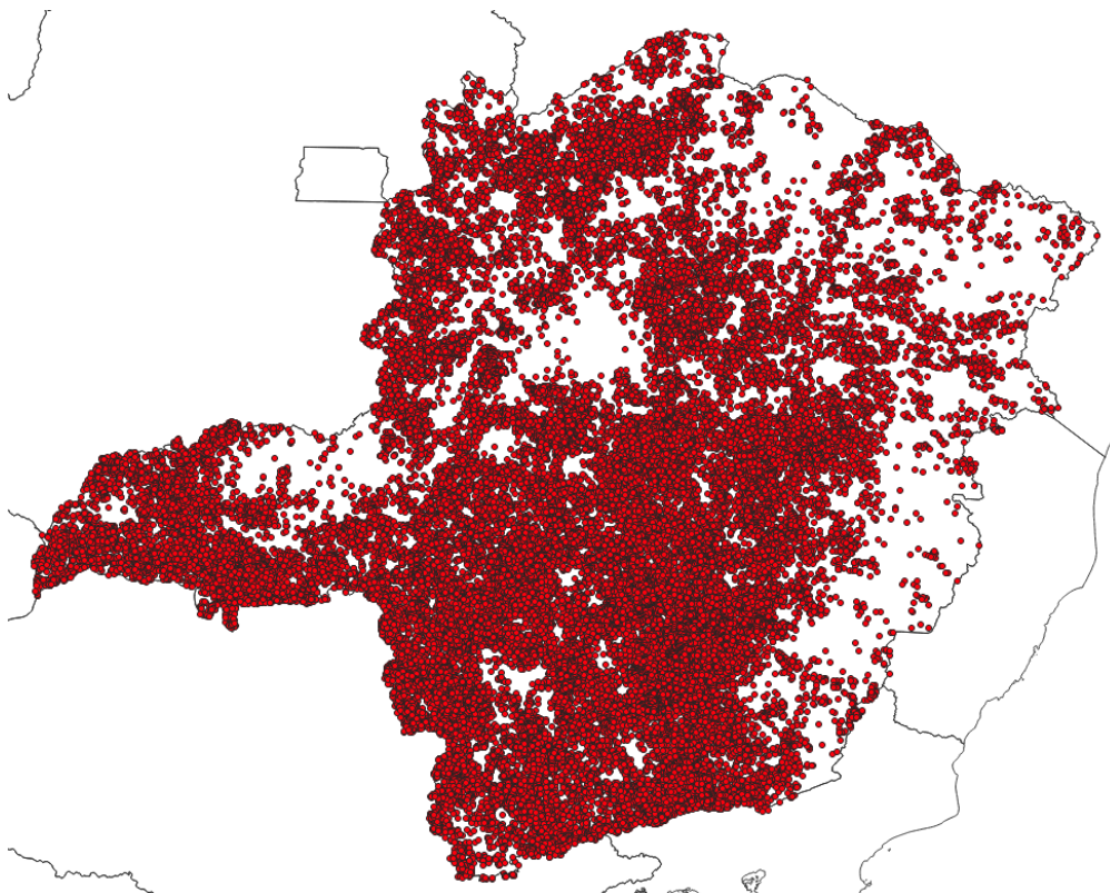
Figura 3 - Localização dos raios registrados entre os dias 28/11 e 02/12 de 2022. Fonte: RINDAT
