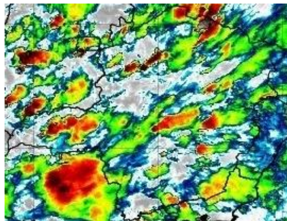
Figura 2 – Seleção de Imagem de Satélite dos dias 28 (a), 29 (b), 30 (c) de novembro e 01 (d) e 02 (e) de dezembro de 2022. Fonte: INPE.
