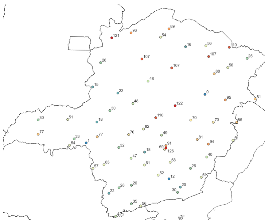
Figura 5b - Pluviometria acumulada entre os dias 10 e 15 de dezembro de 2022. Fonte dos dados: INMET.
