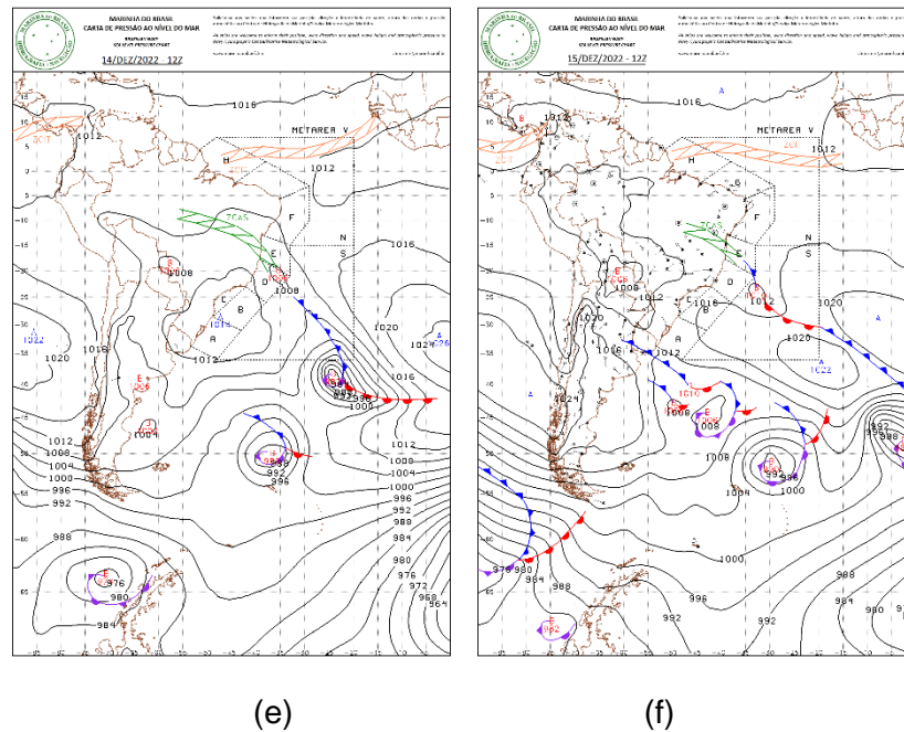
Figura 1 - Carta Sinótica em superfície dos dias 10 (a), 11 (b), 12 (c), 13 (d), 14 (e) e 15 (f) de dezembro de 2022. Fonte: Marinha do Brasil.
