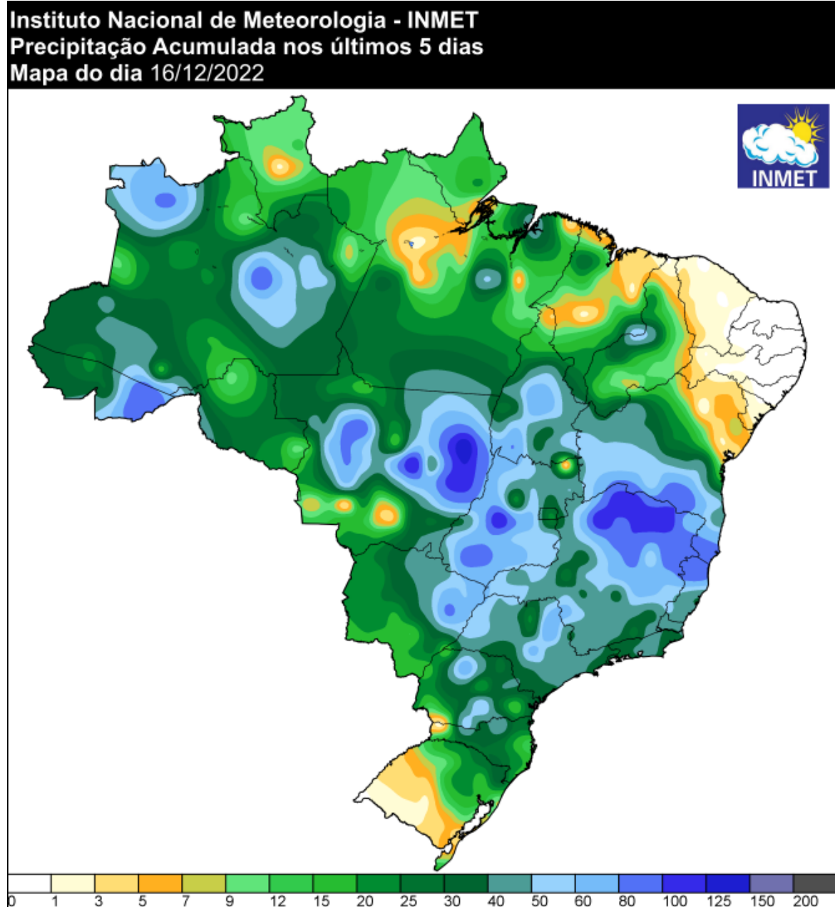
Figura 5a - Pluviometria acumulada (mm) entre os dias 11 e 15 de dezembro de 2022. Fonte: INMET.
