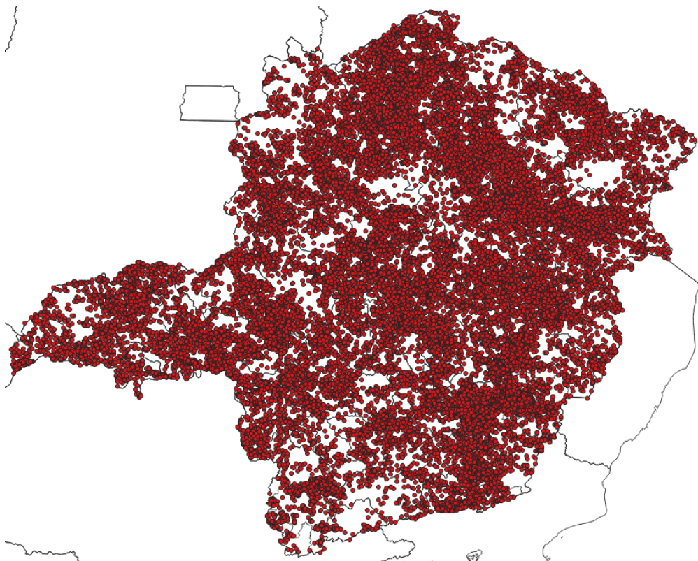
Figura 3 - Localização dos raios registrados entre os dias 10 e 15 de dezembro de 2022. Fonte: RINDAT
