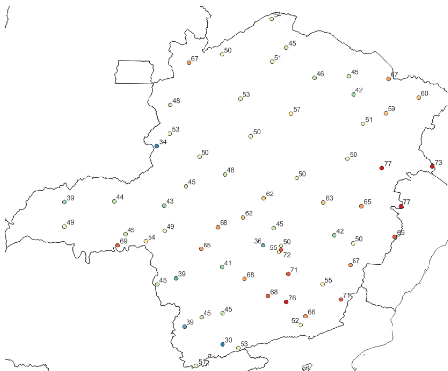
Figura 4 – Rajadas de vento (Km/h) máximas registradas entre os dias 10 e 15 de dezembro de 2022. Fonte: INMET
