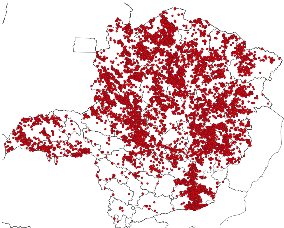
Figura 3 - Localização dos raios registrados entre os dias 04 e 07 de janeiro de 2023. Fonte: RINDAT
