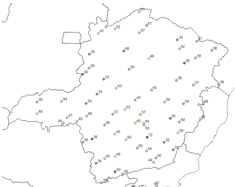
Figura 4 – Rajadas de vento (Km/h) máximas registradas entre os dias 04 e 07 de janeiro de 2023. Fonte: INMET
