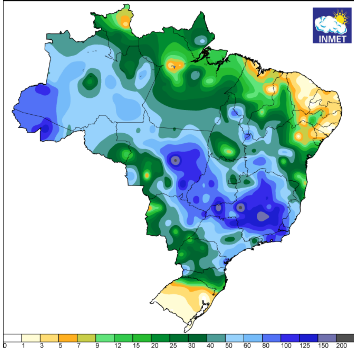
Figura 5a - Pluviometria acumulada (mm) entre os dias 03 e 07 de janeiro de 2023. Fonte: INMET.
