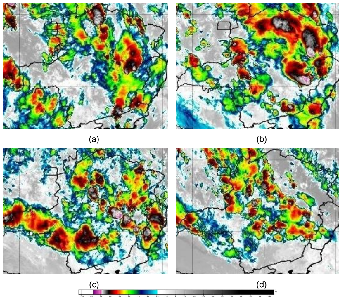
Figura 2 – Seleção de Imagem de Satélite dos dias 04 (a), 05 (b), 06 (c) e 07 (d) de janeiro de 2023. Fonte: INPE.
