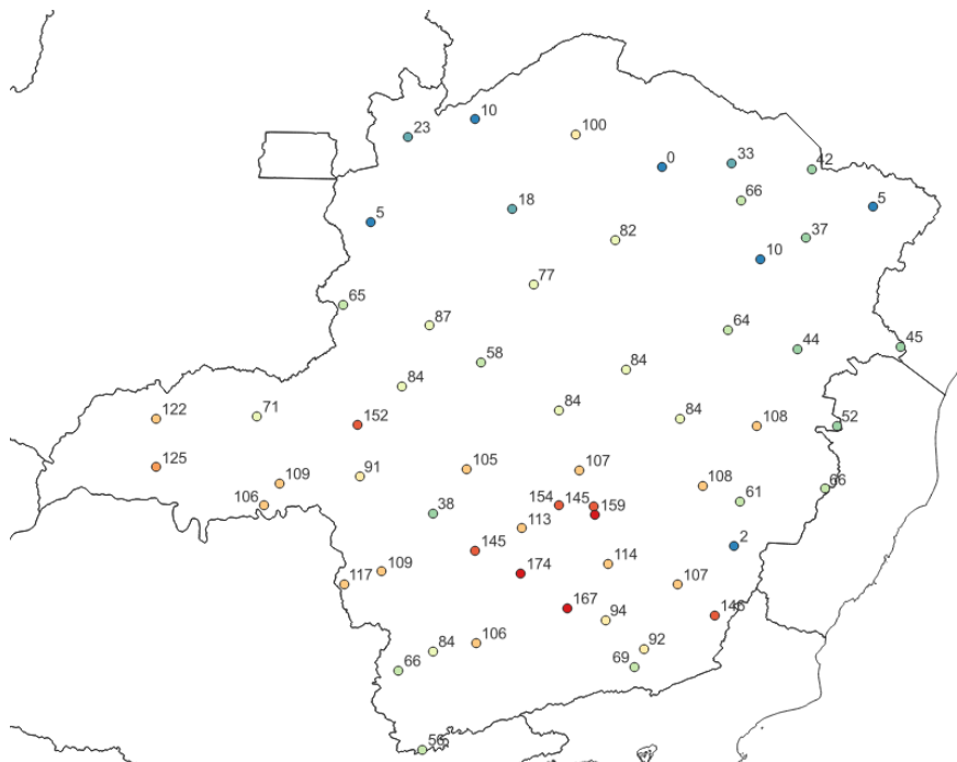
Figura 5b - Pluviometria acumulada entre os dias 04 a 07 de janeiro de 2023. Fonte dos dados: INMET.
