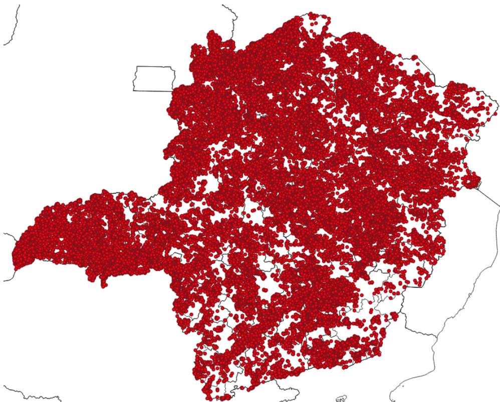
Figura 3 - Localização dos raios registrados entre os dias 19 e 22 de janeiro de 2023. Fonte: RINDAT
