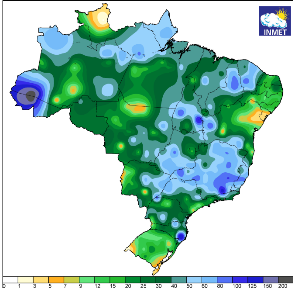
Figura 5a - Pluviometria acumulada (mm) entre os dias 18 e 22 de janeiro de 2023. Fonte: INMET.
