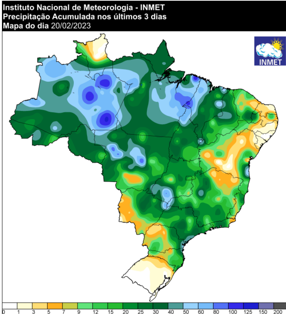
Figura 5a - Pluviometria acumulada (mm) entre os dias 17 e 19 de fevereiro de 2023. Fonte: INMET.
