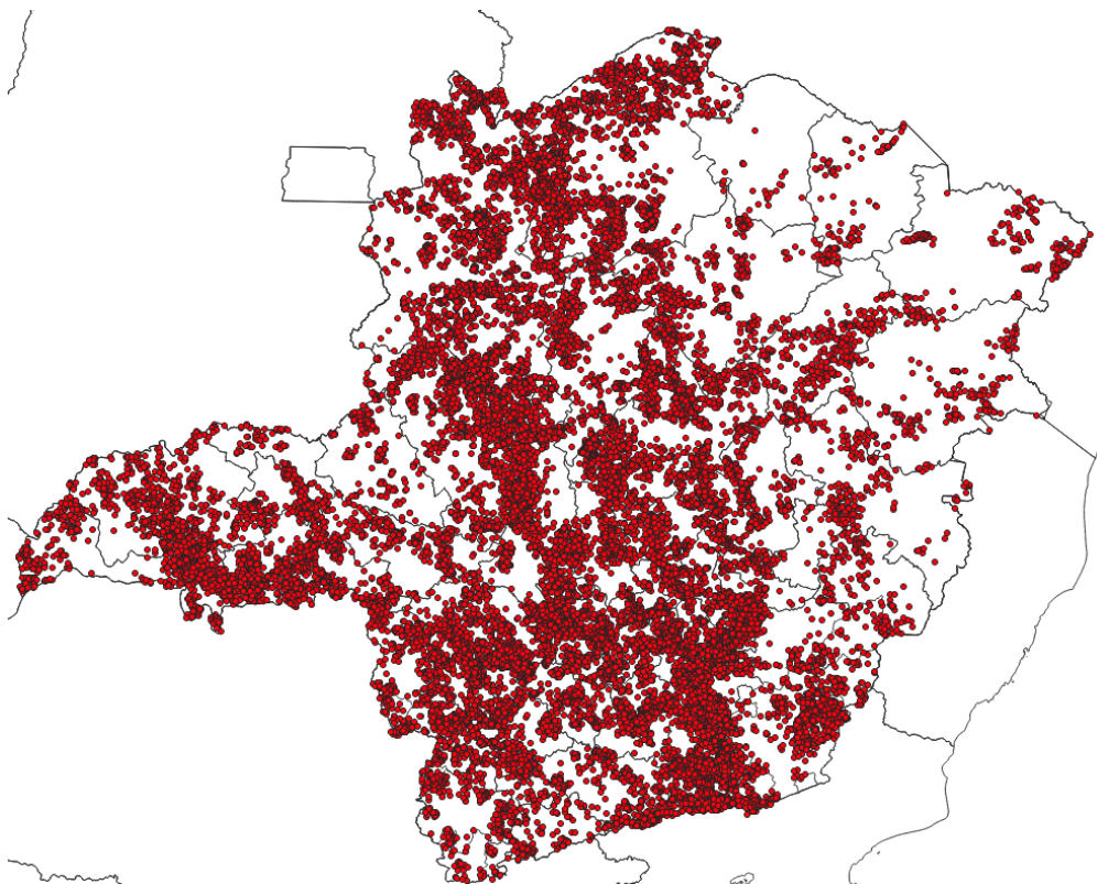
Figura 3 - Localização dos raios registrados entre os dias 17 e 19 de fevereiro de 2023. Fonte: RINDAT
