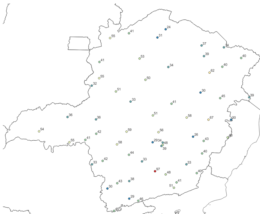
Figura 4 – Rajadas de vento (Km/h) máximas registradas entre os dias 17 e 19 de fevereiro de 2023. Fonte: INMET
