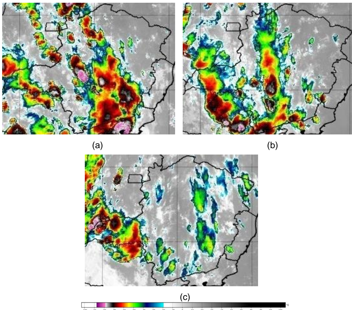
Figura 2 – Seleção de Imagem de Satélite dos dias 17 (a), 18 (b) e 19 (c) de fevereiro de 2023. Fonte: INPE.
