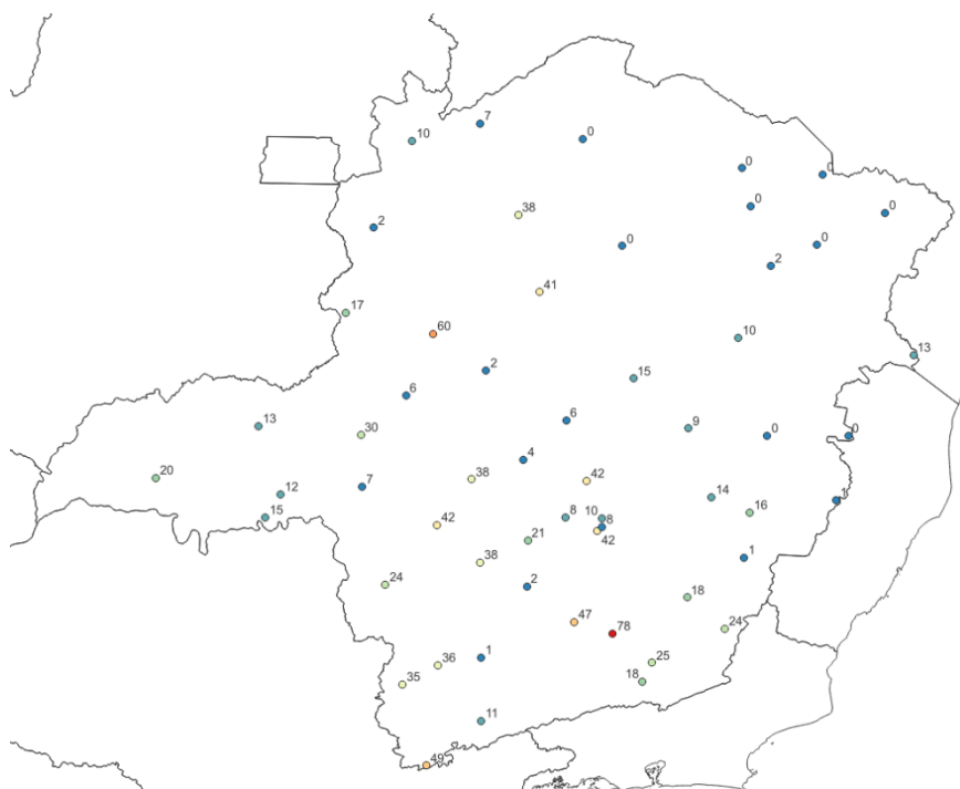
Figura 5b - Pluviometria acumulada entre os dias 17 a 19 de fevereiro de 2023. Fonte dos dados: INMET.
