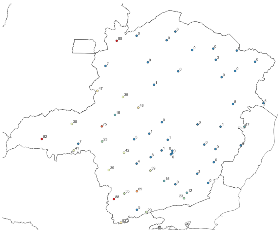
Figura 5b - Pluviometria acumulada entre os dias 05 e 08 de março de 2023. Fonte dos dados: INMET.
