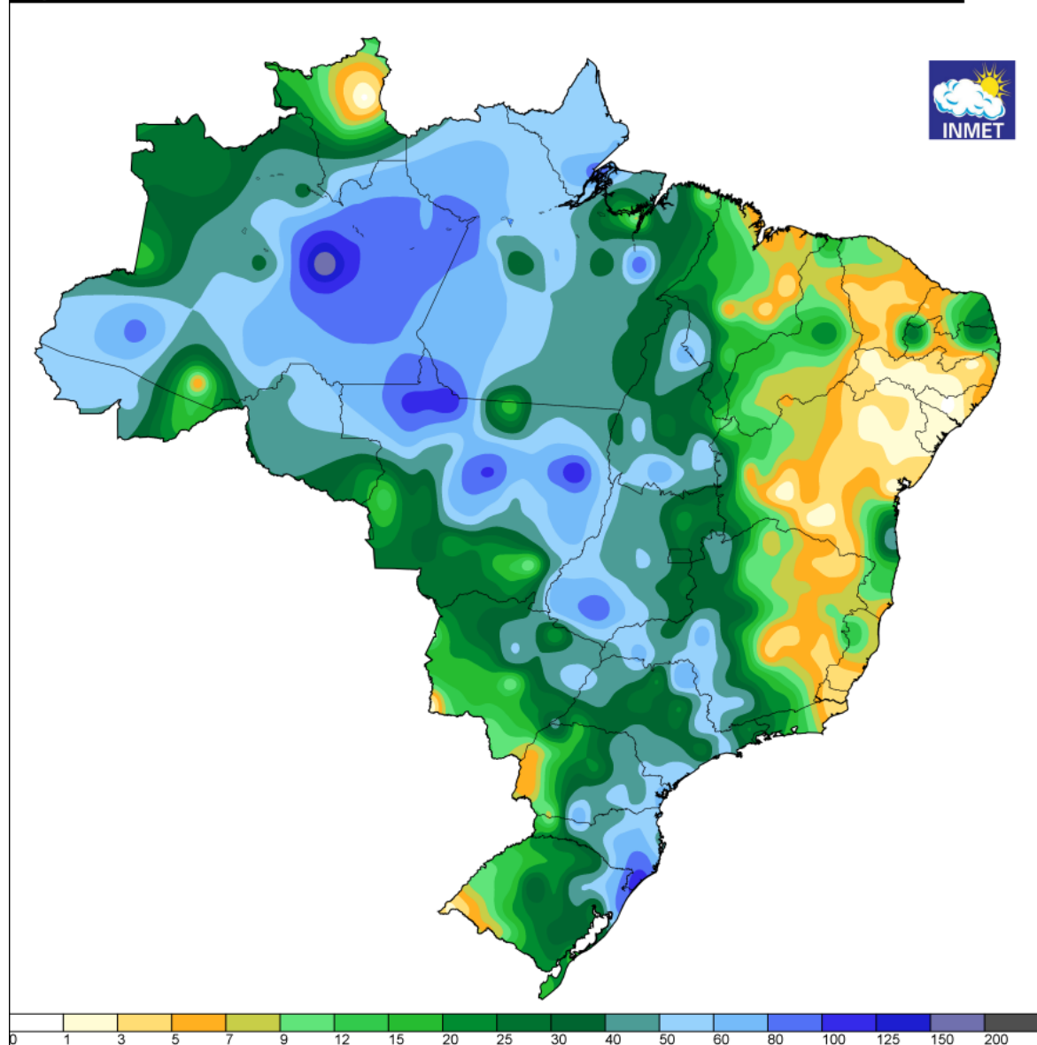
Figura 5a - Pluviometria acumulada (mm) entre os dias 04 e 08 de março de 2023. Fonte: INMET.
