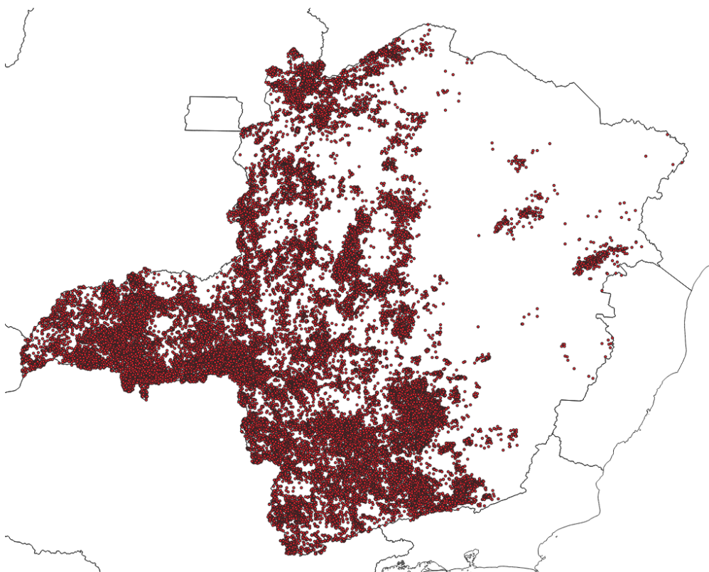
Figura 3 - Localização dos raios registrados entre os dias 05 e 08 de março de 2023. Fonte: RINDAT
