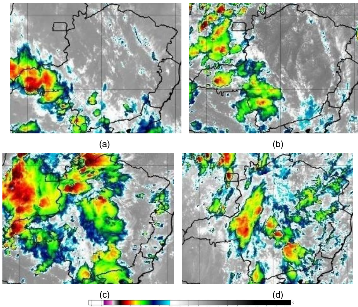
Figura 2 – Seleção de Imagem de Satélite dos dias 05 (a), 06 (b), 07 (c) e 08 (d) de março de 2023. Fonte: INPE.
