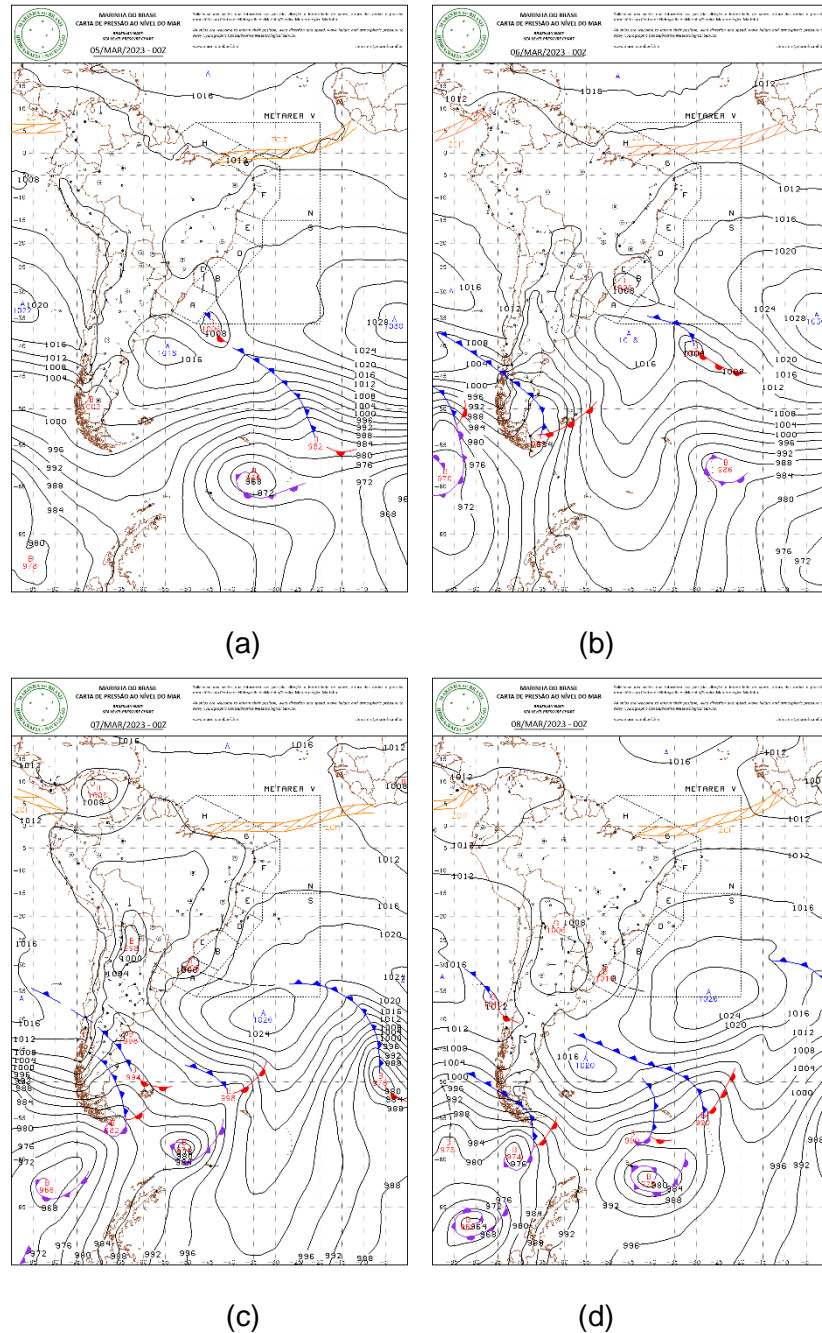
Figura 1 - Carta Sinótica em superfície dos dias 05 (a), 06 (b), 07 (c) e 08 (d) de março de 2023. Fonte: Marinha do Brasil.
