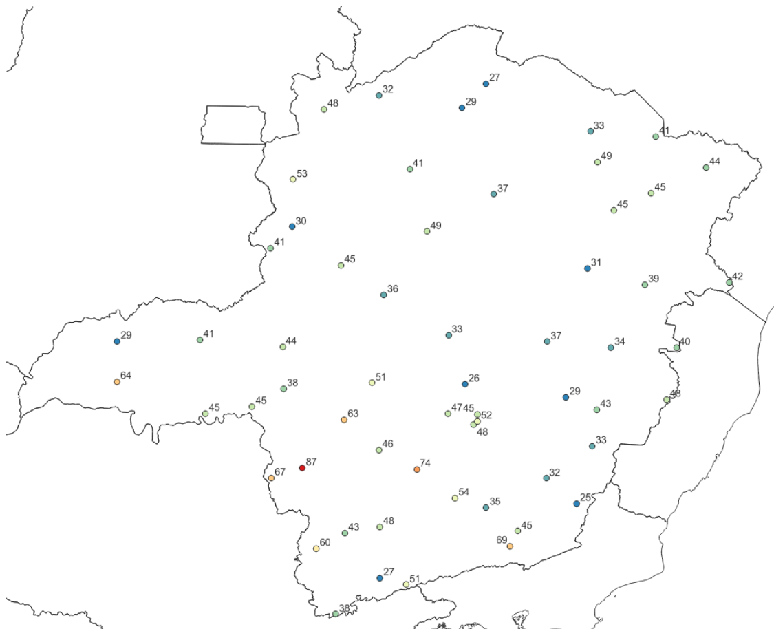
Figura 4 – Rajadas de vento (Km/h) máximas registradas entre os dias 05 e 08 de março de 2023. Fonte: INMET
