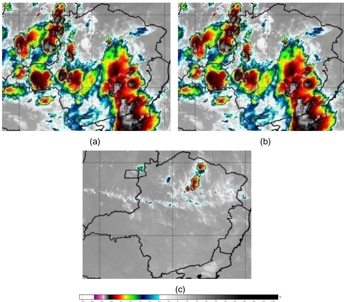
Figura 2 – Seleção de Imagem de Satélite dos dias 14 (a), 15 (b) e 16 (c) de abril de 2023. Fonte: INPE.
