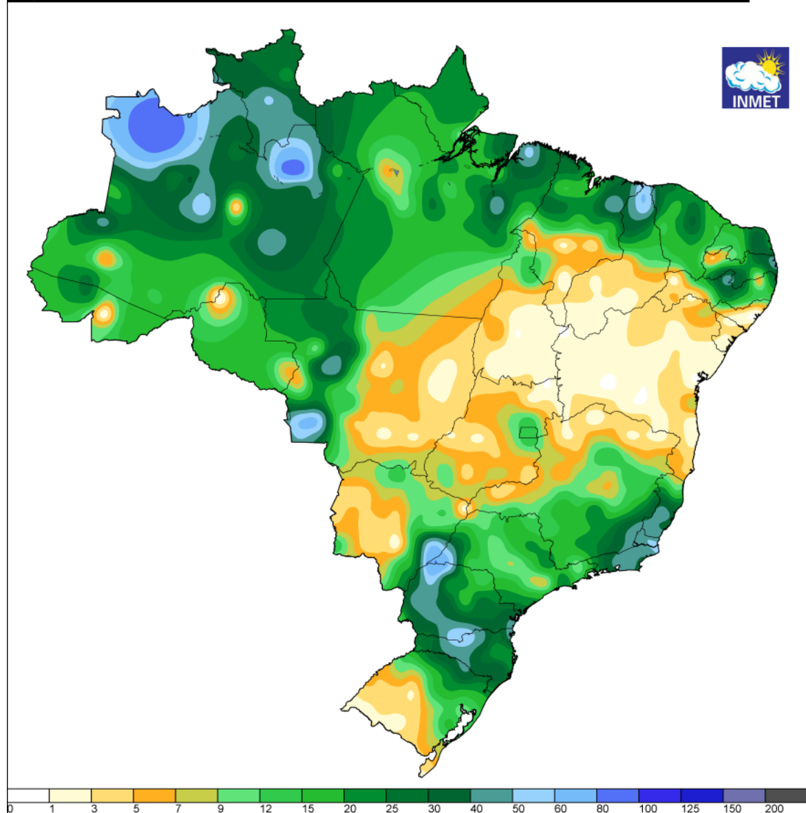
Figura 5a - Pluviometria acumulada (mm) entre os dias 14 e 16 de abril de 2023. Fonte: INMET.
