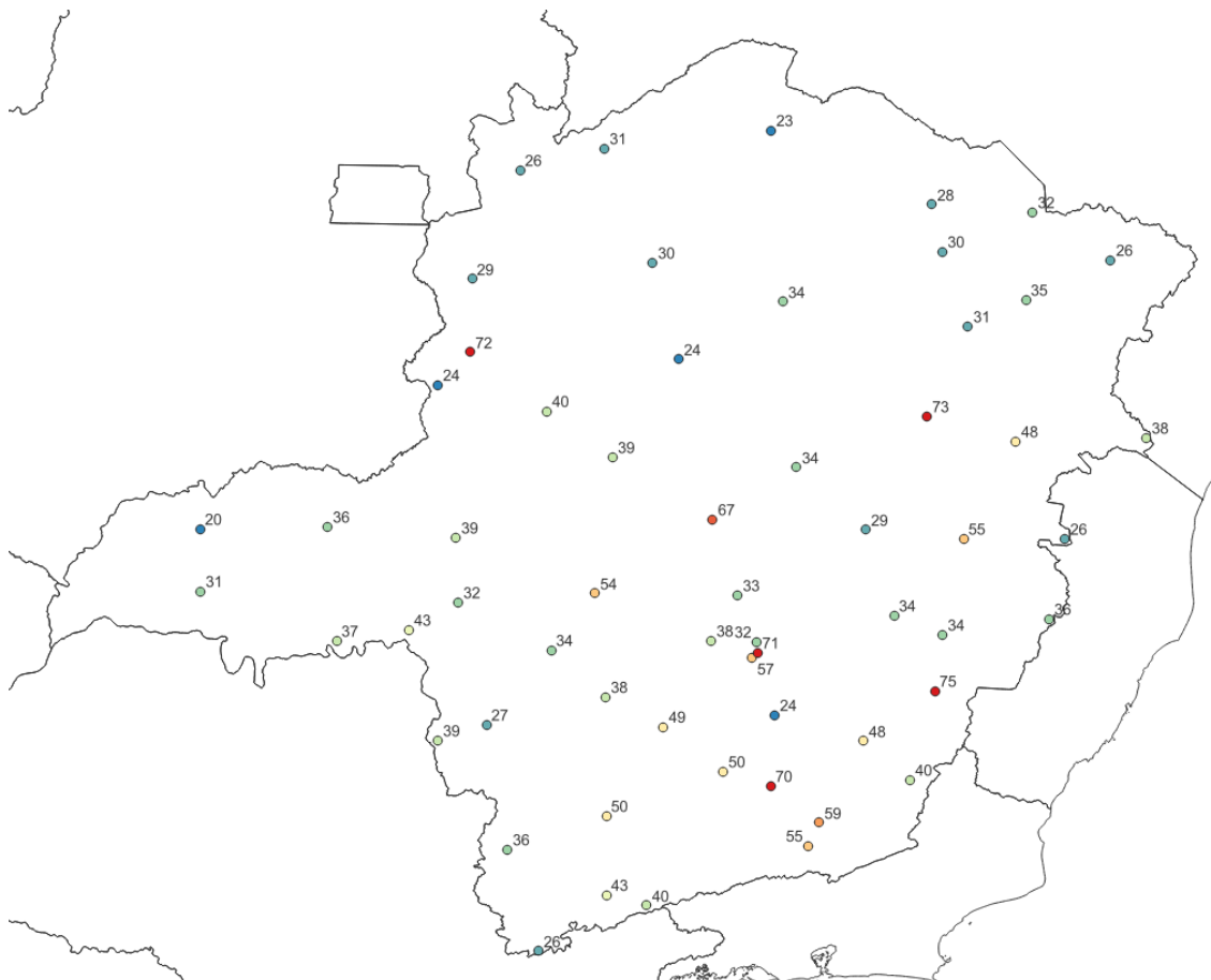
Figura 4 – Rajadas de vento (Km/h) máximas registradas entre os dias 14 e 16 de abril de 2023. Fonte: INMET
