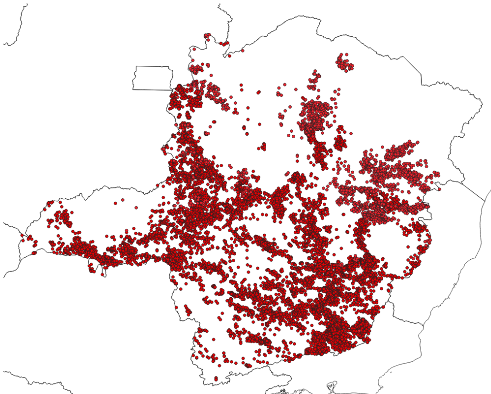
Figura 3 - Localização dos raios registrados entre os dias 14 e 16 de abril de 2023. Fonte: RINDAT
