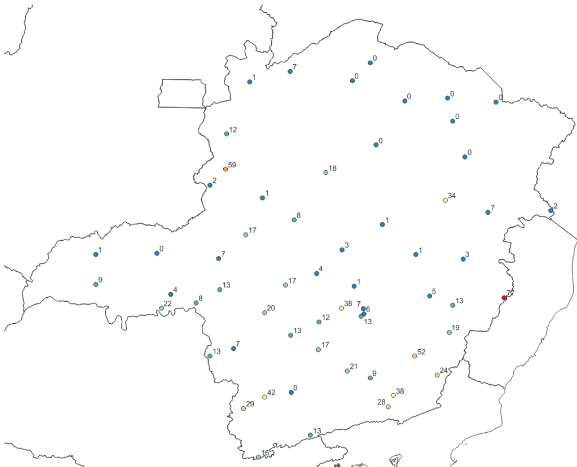
Figura 5b - Pluviometria acumulada entre os dias 14 e 16 de abril de 2023. Fonte dos dados: INMET.
