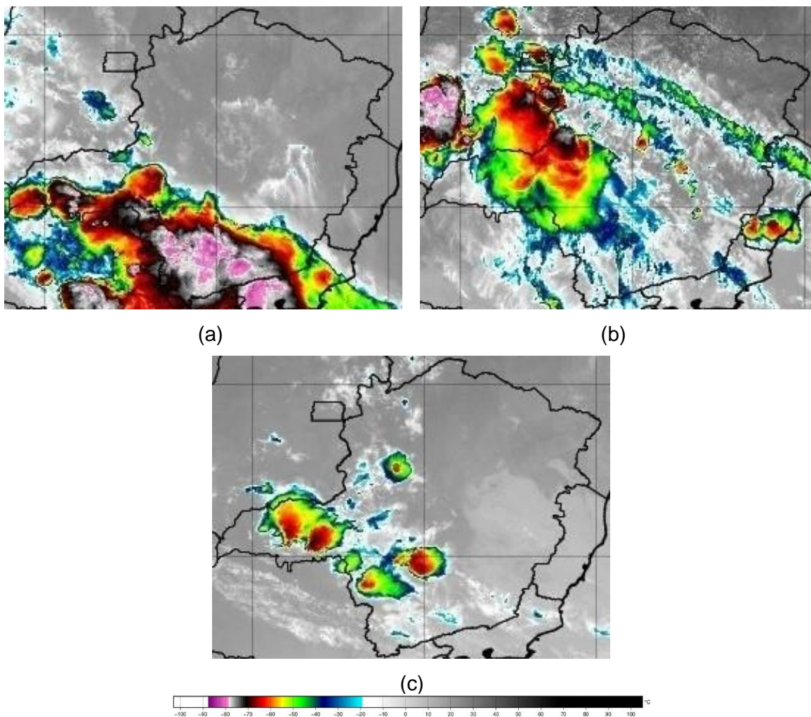
Figura 2 – Seleção de Imagem de Satélite dos dias 12 (a), 13 (b) e 14 (c) de outubro de 2023. Fonte: INPE.
