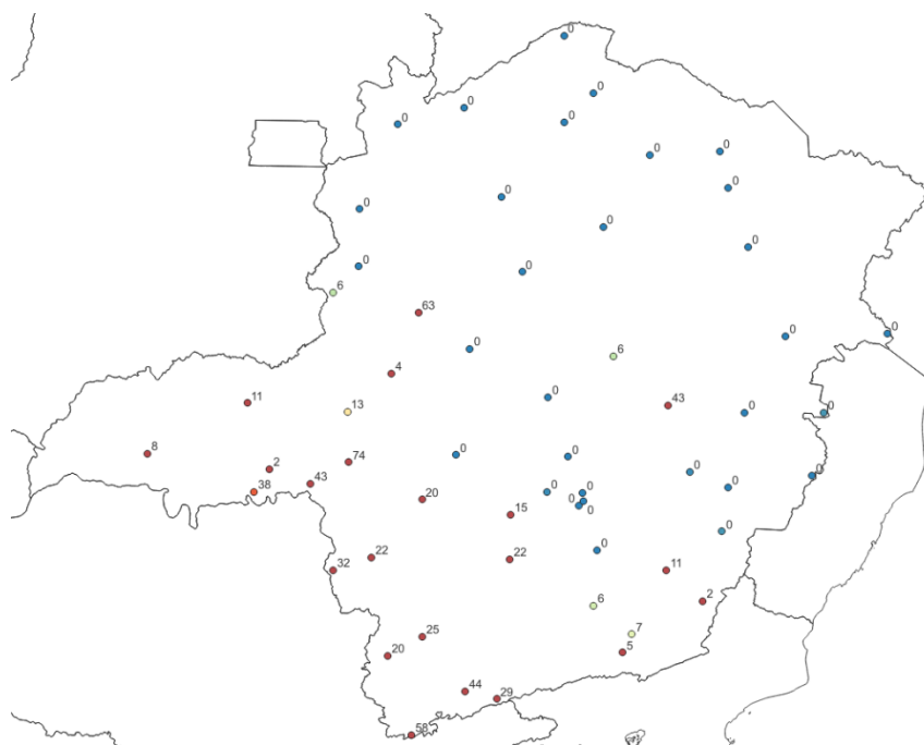
Figura 5b - Pluviometria acumulada entre os dias 12 e 14 de outubro de 2023. Fonte dos dados: INMET.
