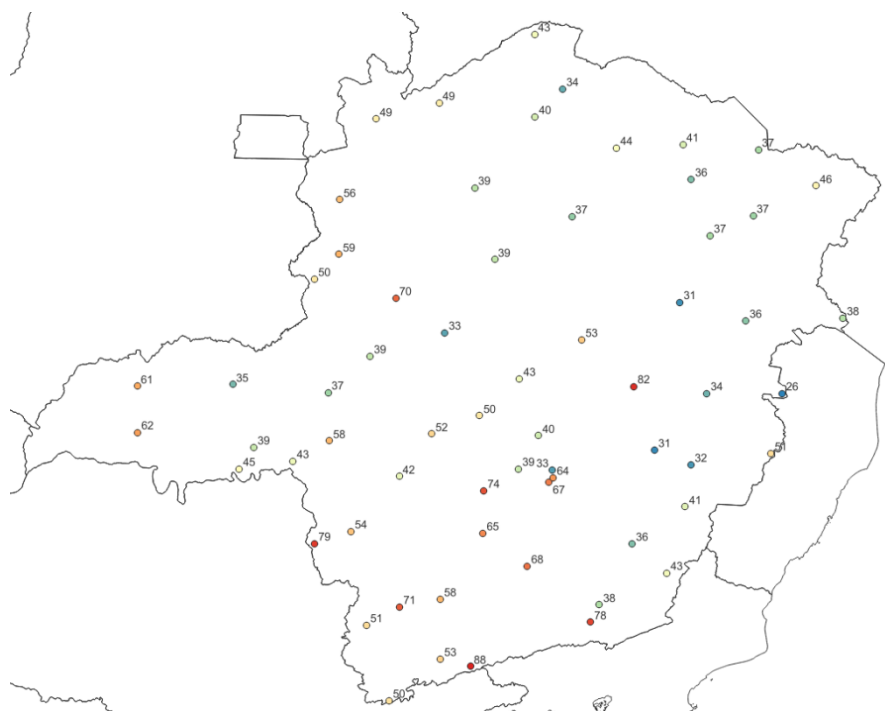
Figura 4 – Rajadas de vento (Km/h) máximas registradas entre os dias 12 e 14 de outubro de 2023. Fonte: INMET
