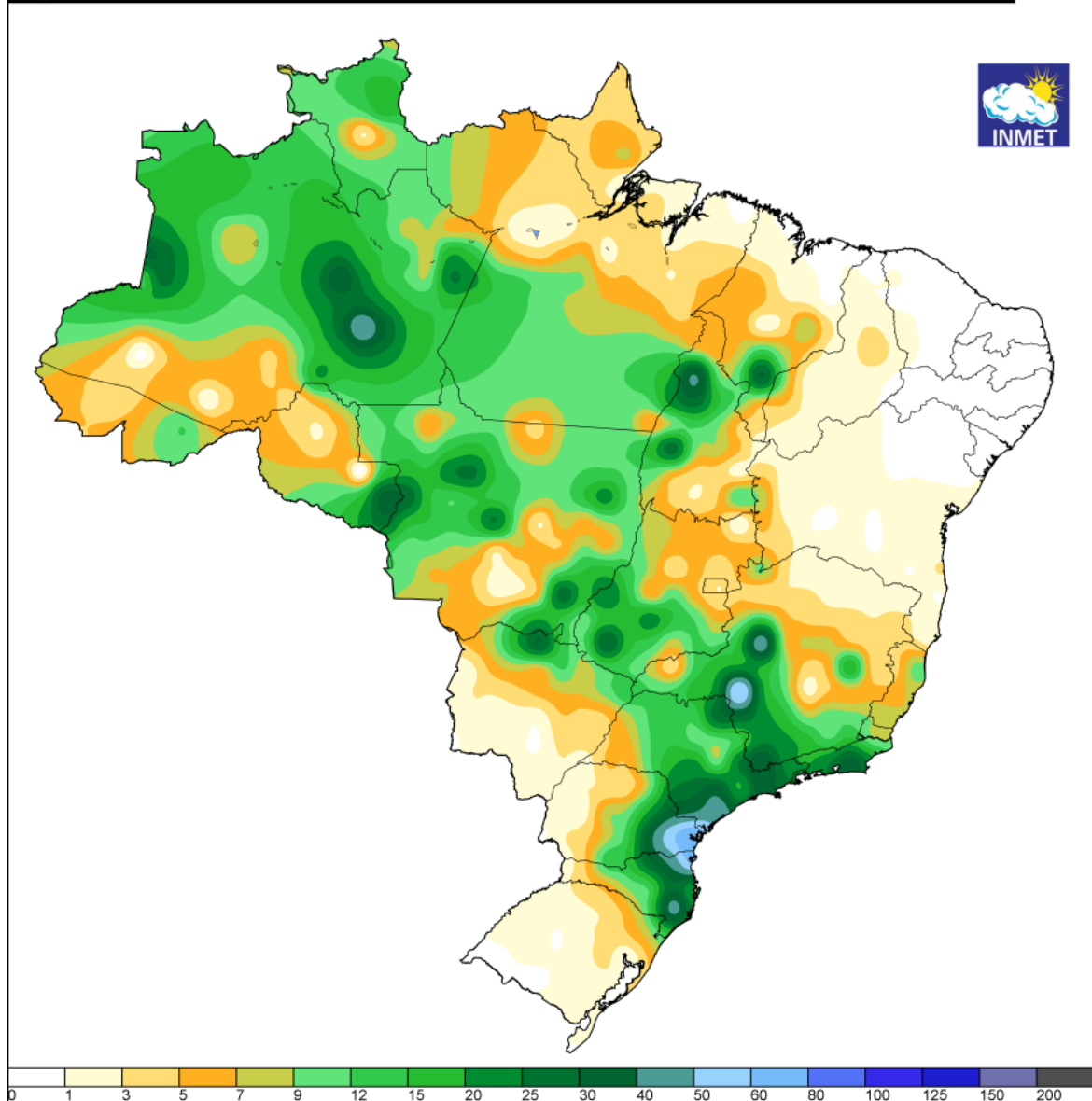
Figura 5a - Pluviometria acumulada (mm) entre os dias 12 e 14 de outubro de 2023. Fonte: INMET.
