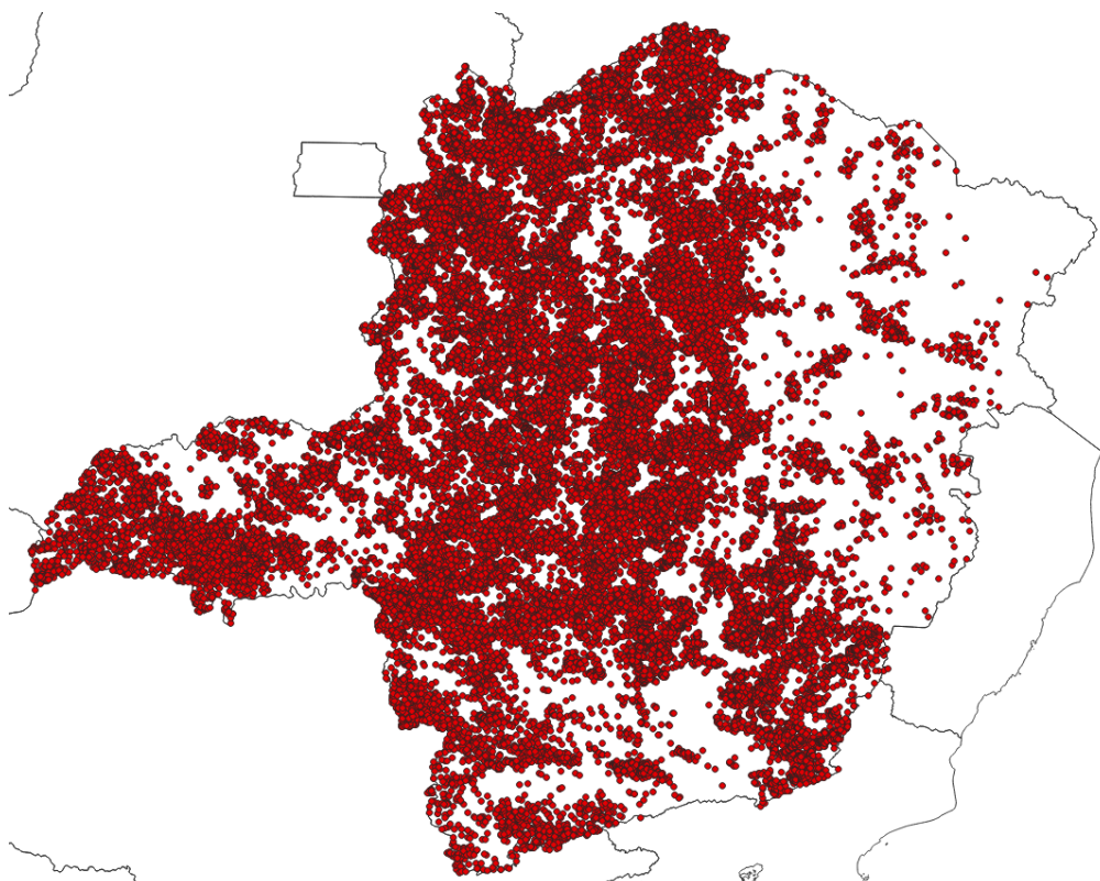
Figura 3 - Localização dos raios registrados entre os dias 01 e 04 de novembro de 2023. Fonte: RINDAT
