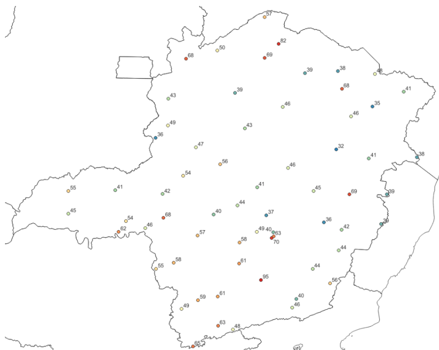
Figura 4 – Rajadas de vento (Km/h) máximas registradas entre os dias 01 e 04 de novembro de 2023. Fonte: INMET
