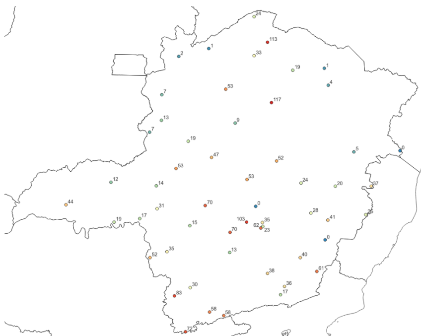
Figura 5b - Pluviometria acumulada entre os dias 01 e 04 de novembro de 2023. Fonte dos dados: INMET.
