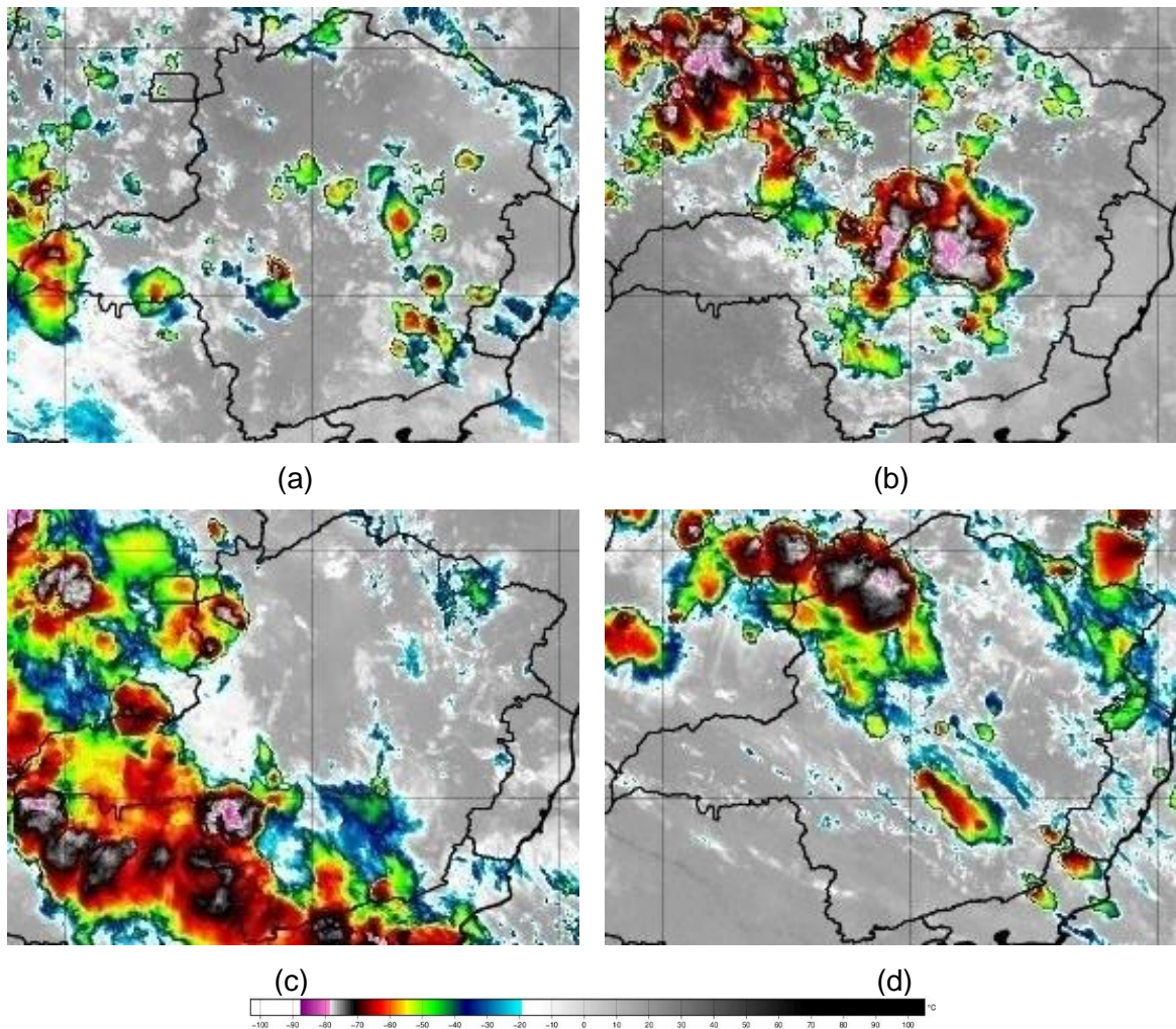
Figura 2 – Seleção de Imagens de Satélite dos dias 01 (a), 02 (b), 03 (c) e 04 (d) de novembro de 2023. Fonte: INPE.
