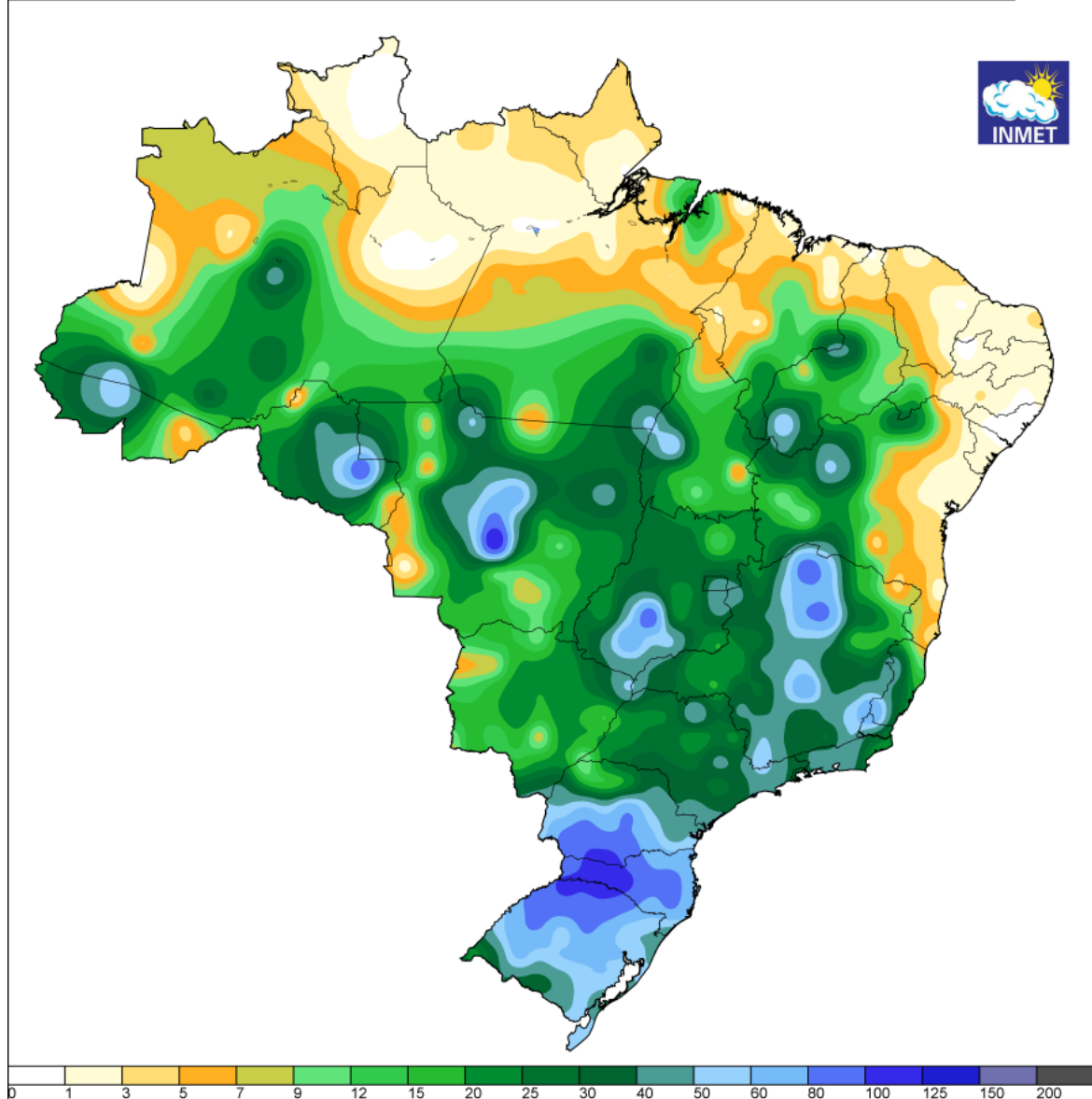
Figura 5a - Pluviometria acumulada (mm) entre os dias 31 de outubro e 04 de novembro de 2023. Fonte: INMET.
