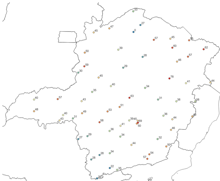
Figura 4 – Rajadas de vento (Km/h) máximas registradas entre os dias 01 e 03 de dezembro de 2023. Fonte: INMET
