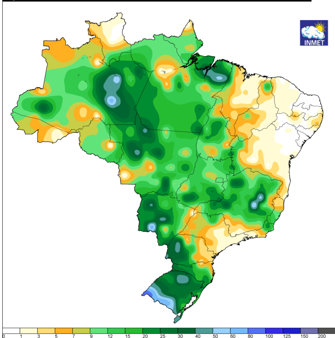
Figura 5a - Pluviometria acumulada (mm) entre os dias 01 e 03 de dezembro de 2023. Fonte: INMET.
