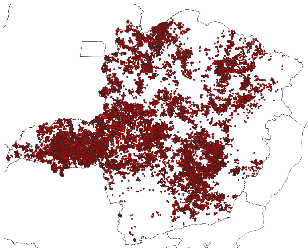
Figura 3 - Localização dos raios registrados entre os dias 01 e 03 de dezembro de 2023. Fonte: RINDAT
