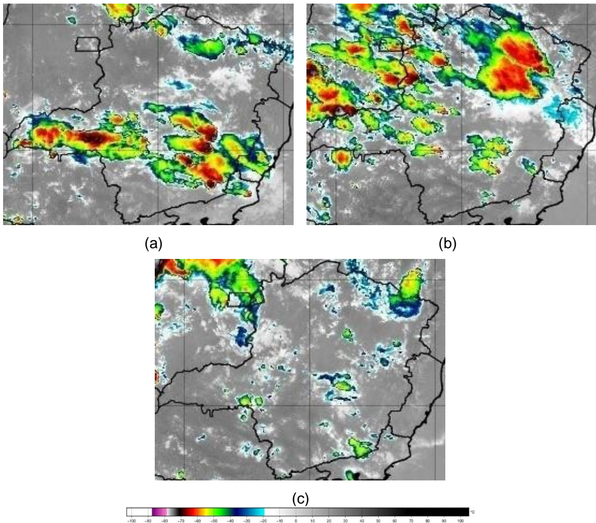
Figura 2 – Seleção de Imagem de Satélite dos dias 01 (a), 02 (b) e 03 (c) de dezembro de 2023. Fonte: INPE.
