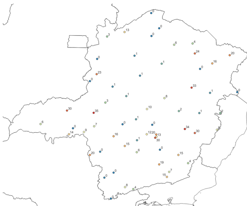
Figura 5b - Pluviometria acumulada entre os dias 01 e 03 de dezembro de 2023. Fonte dos dados: INMET.
