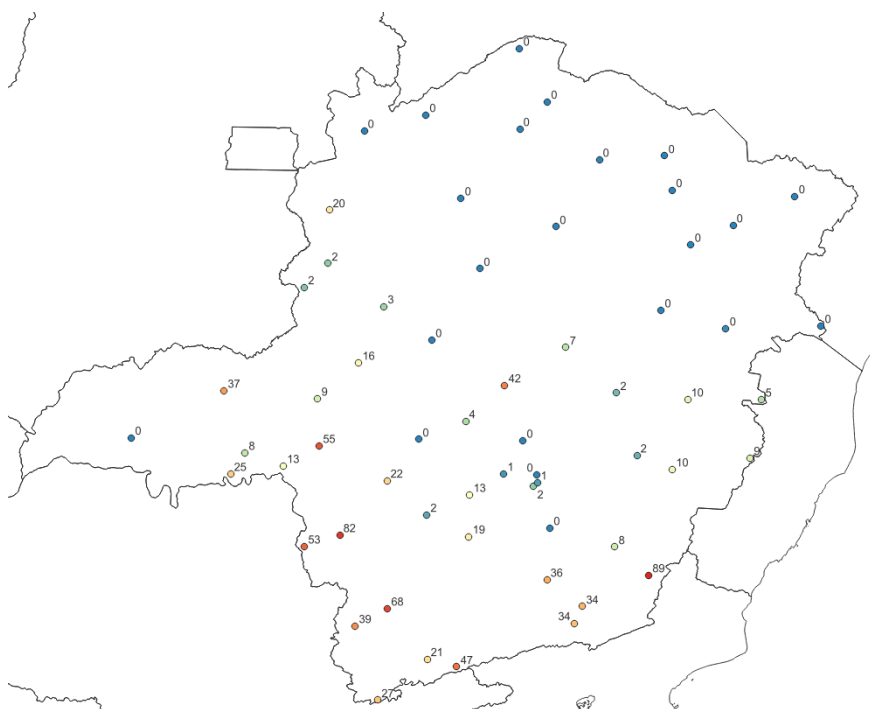
Figura 5b - Pluviometria acumulada entre os dias 08 e 12 de dezembro de 2023. Fonte dos dados: INMET.
