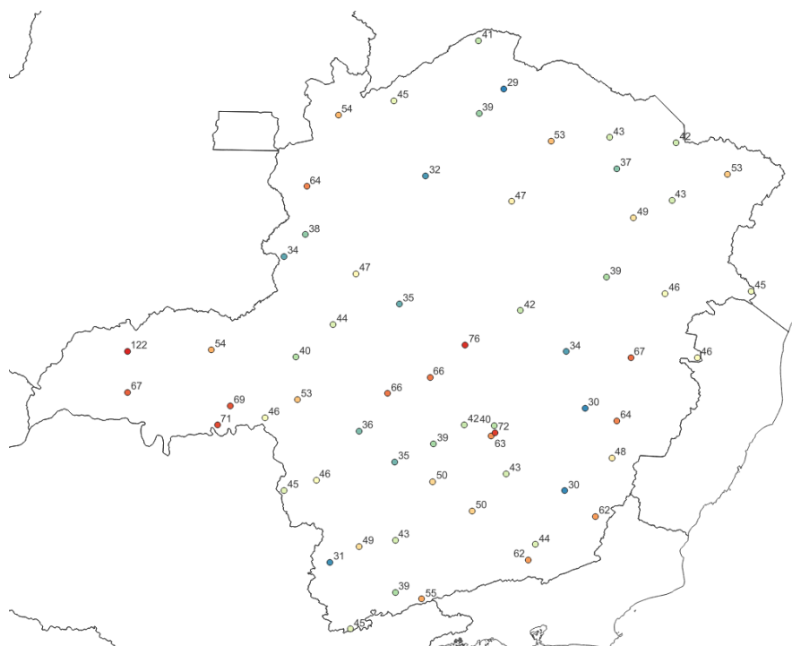
Figura 4 – Rajadas de vento (Km/h) máximas registradas entre os dias 08 e 12 de dezembro de 2023. Fonte: INMET
