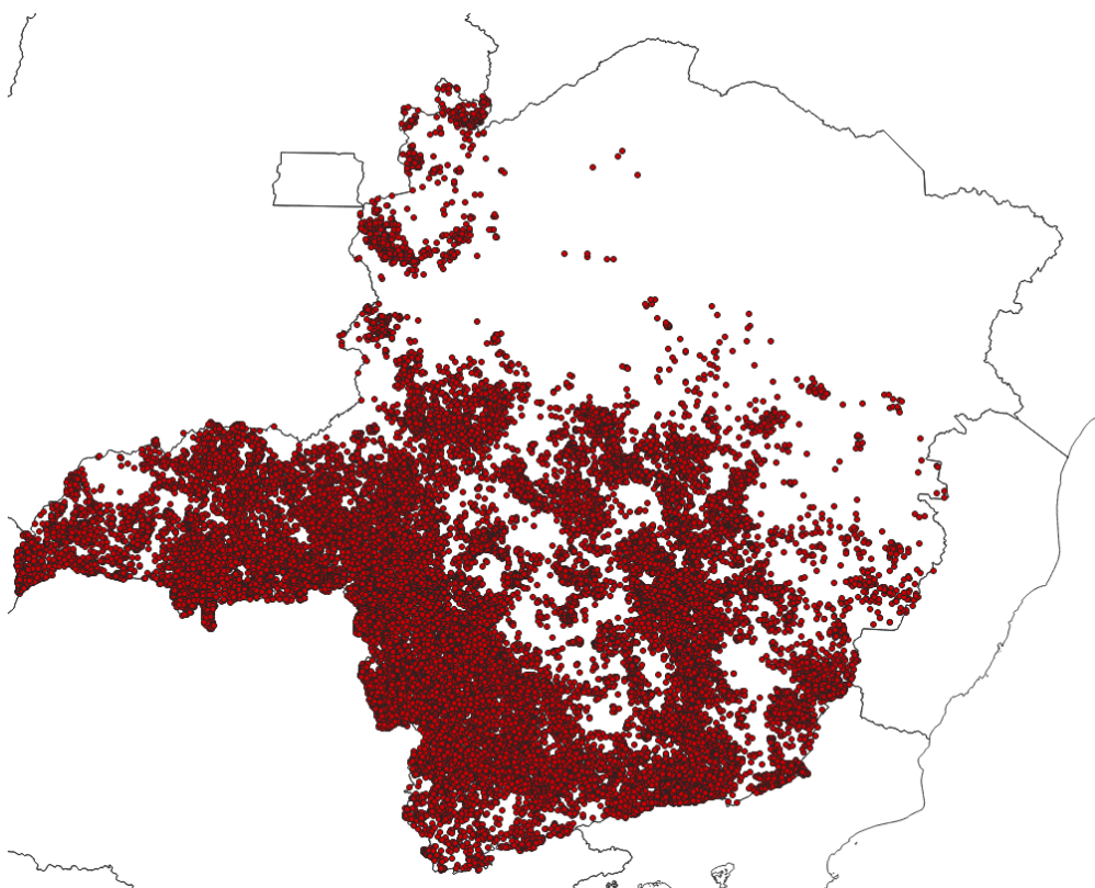
Figura 3 - Localização dos raios registrados entre os dias 08 e 12 de dezembro de 2023. Fonte: RINDAT
