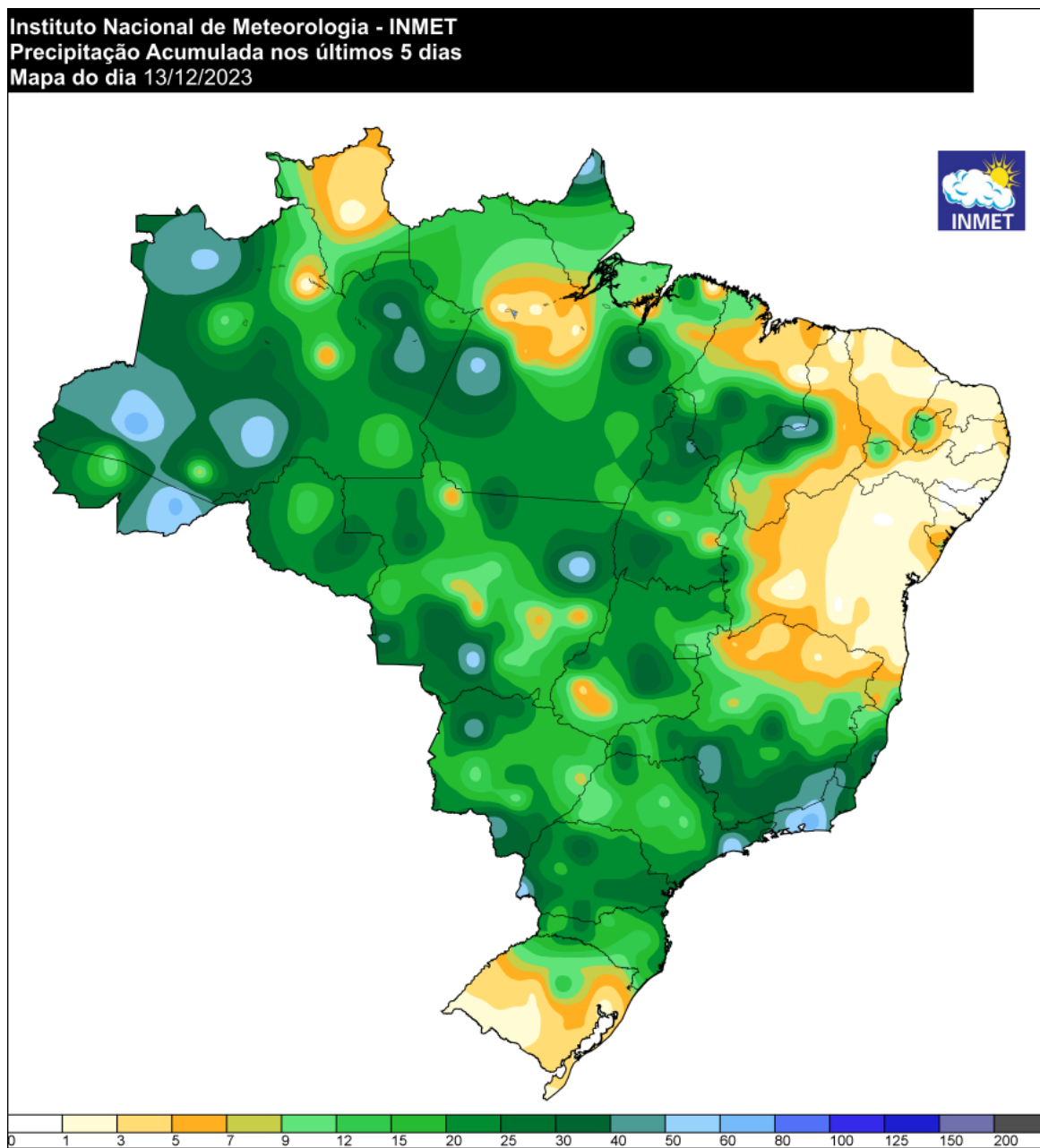
Figura 5a - Pluviometria acumulada (mm) entre os dias 08 e 12 de dezembro de 2023. Fonte: INMET.
