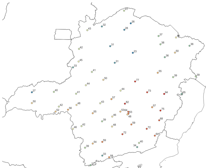
Figura 4 – Rajadas de vento (Km/h) máximas registradas entre os dias 25 e 27 de dezembro de 2023. Fonte: INMET
