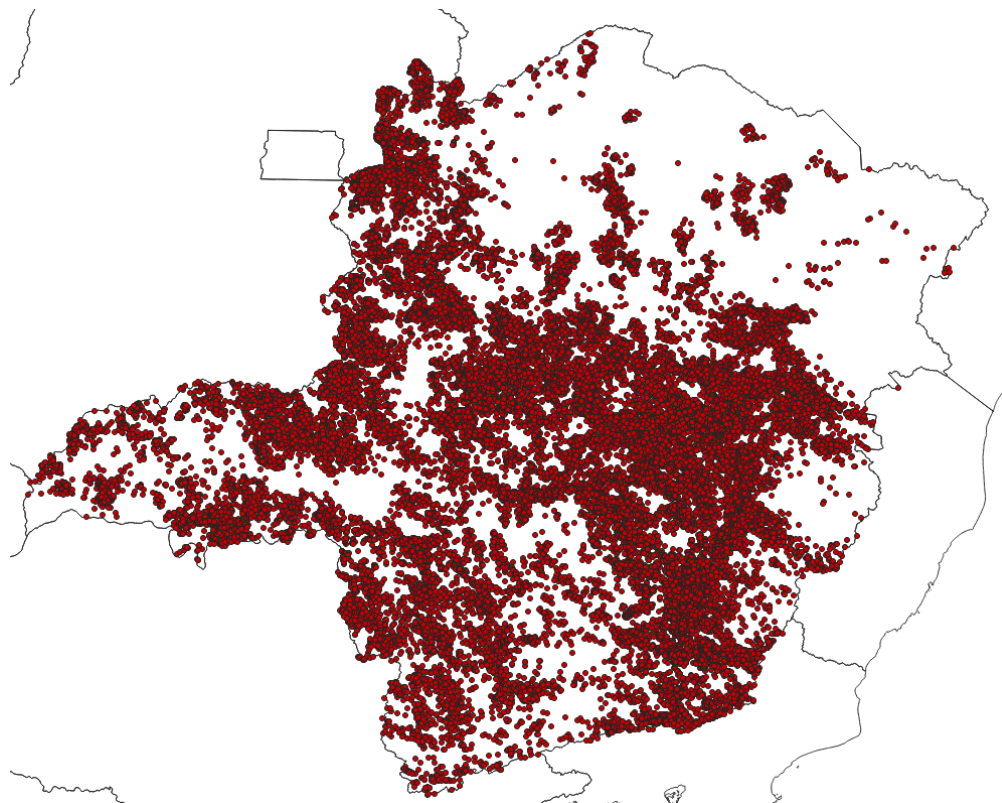
Figura 3 - Localização dos raios registrados entre os dias 25 e 27 de dezembro de 2023. Fonte: RINDAT
