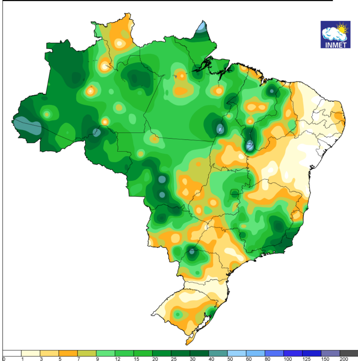
Figura 5a - Pluviometria acumulada (mm) entre os dias 25 e 27 de dezembro de 2023. Fonte: INMET.
