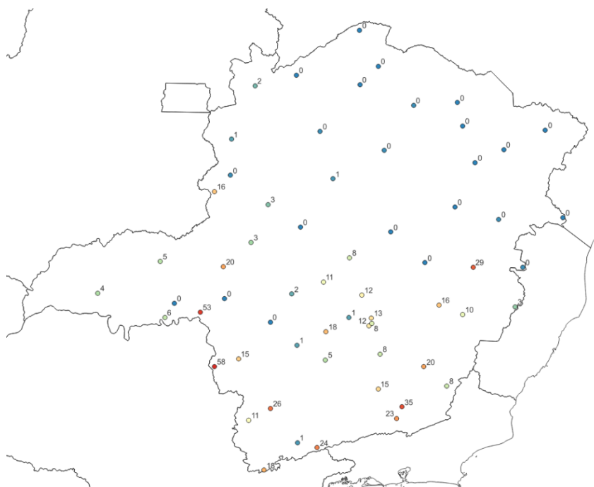
Figura 5b - Pluviometria acumulada entre os dias 25 e 27 de dezembro de 2023. Fonte dos dados: INMET.
