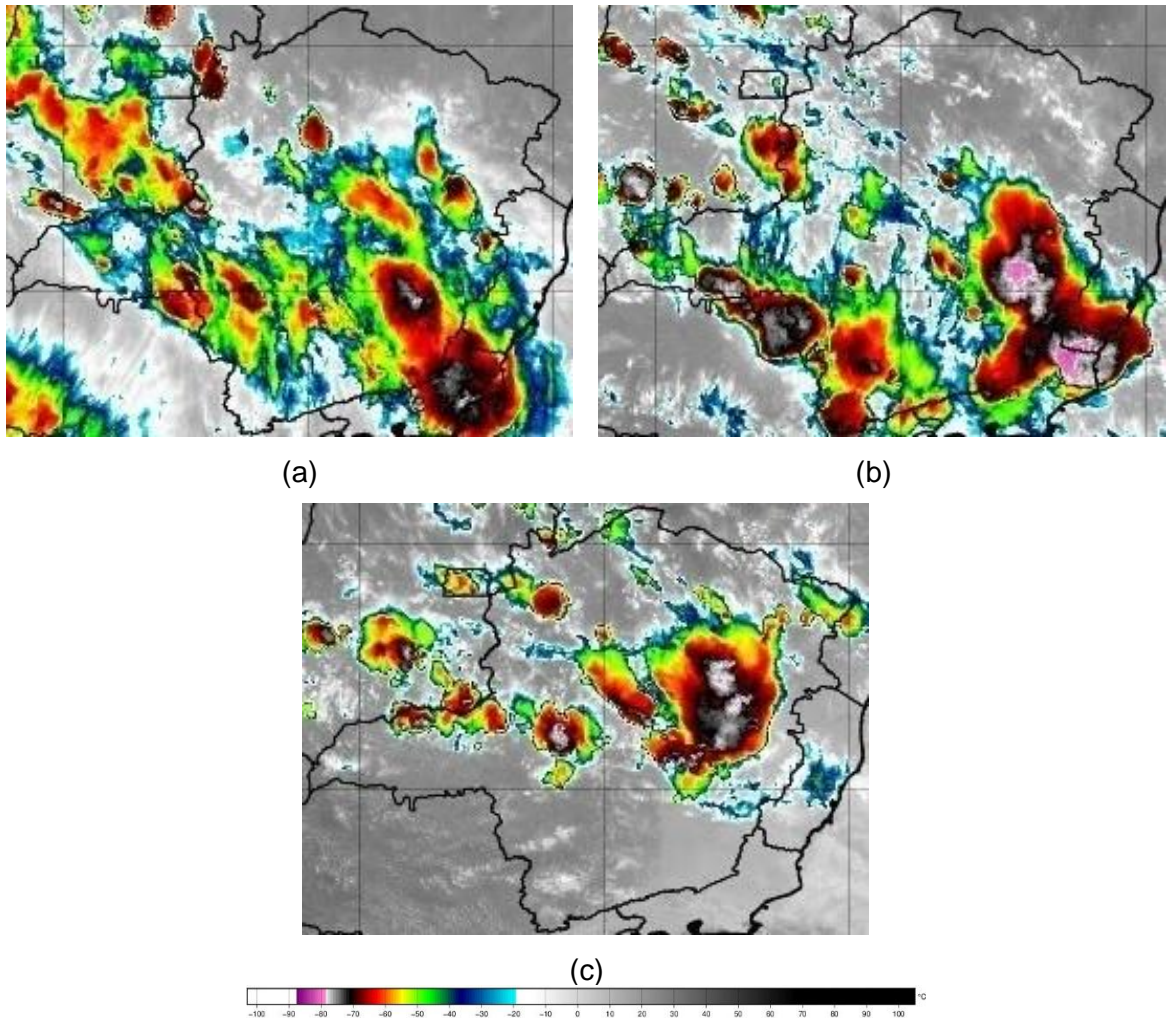
Figura 2 – Seleção de Imagem de Satélite dos dias 25 (a), 26 (b) e 27 (c) de dezembro de 2023. Fonte: INPE.
