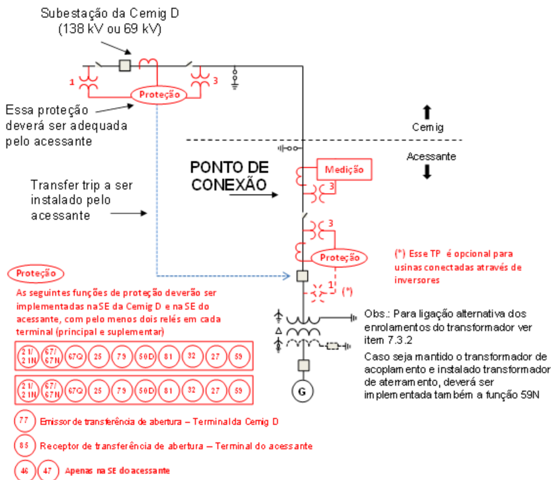
Figura 8 - Consumidor que pretende se tornar autoprodutor (Ligado na extremidade de linha)
