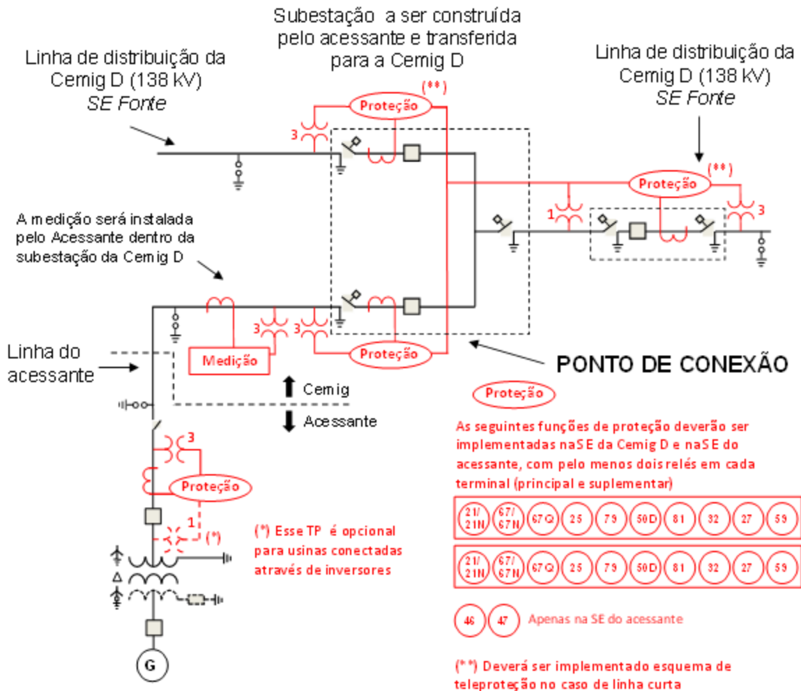
Figura 5 – Subestação de integração de 138 kV – Sistema em anel
