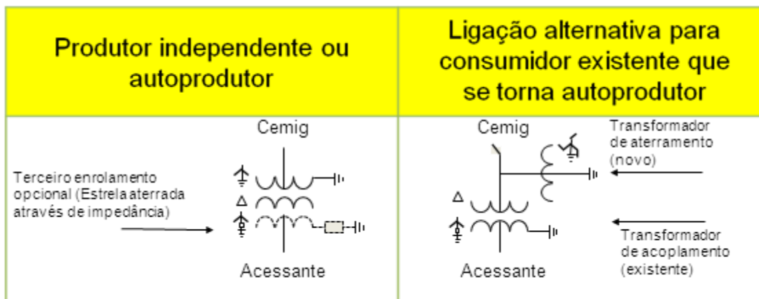
Figura 10 - ligação de Transformador de Acoplamento
