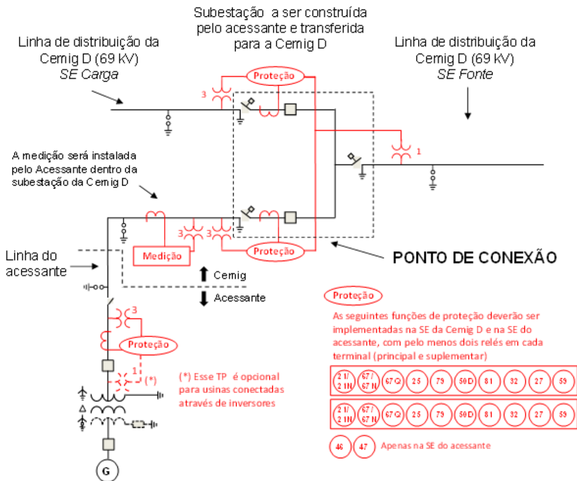
Figura 4 – SE de integração de 69 kV
